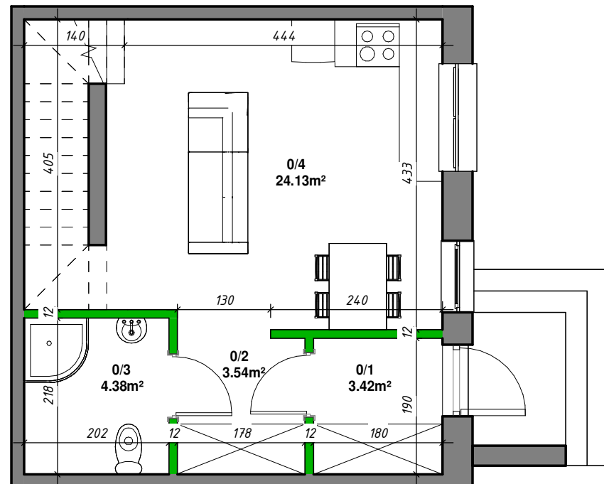
Rzut parteru
