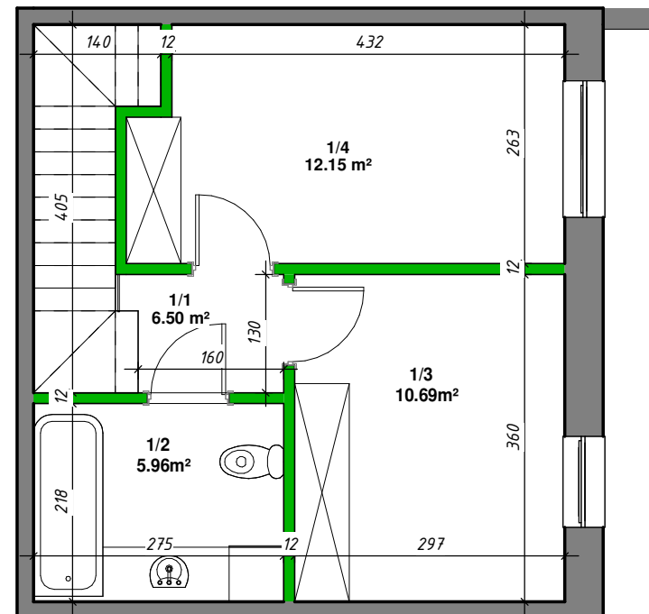
Rzut piętra
