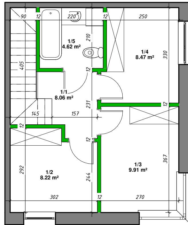
Rzut piętra
