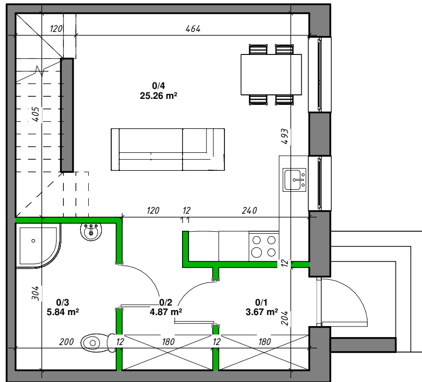
Rzut parteru
