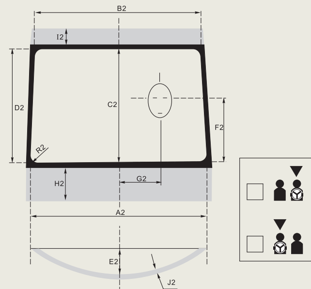
Windshield Model Drawing 玻璃模型图
