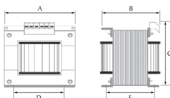
TES | Transformer
