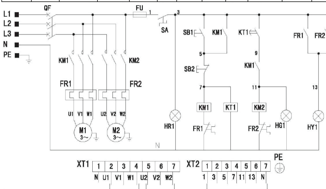
Exhaust fan Supply fan Connection
