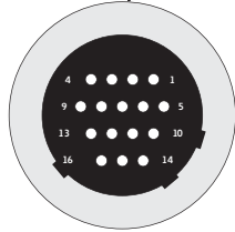
Main Male Connector Ana Erkek Konnektörü
