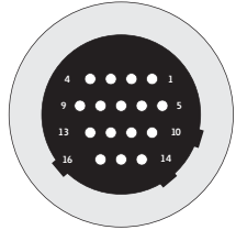
Main Male Connector Ana Erkek Konnektörü
