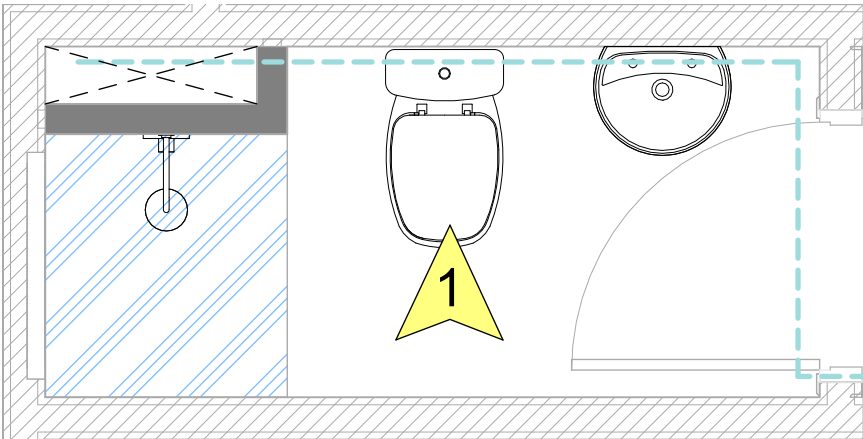
PLANTA
