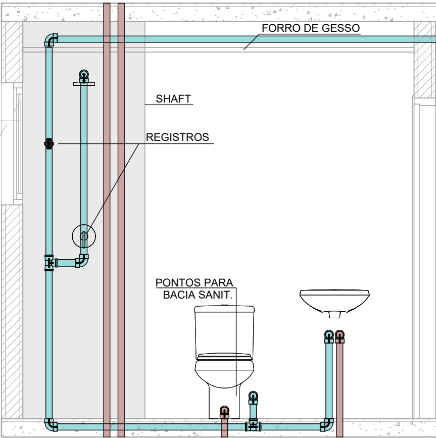
VISTA 1
