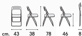
articolo 2078 sedia pieghevole struttura in metallo e seduta in polipropilene colore nero. chair with metal structure and seat in black color polypropylene.
