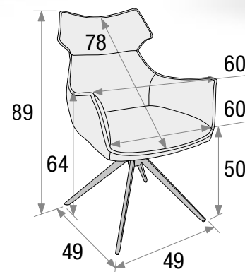
articolo 2344 Poltrona girevole struttura metallo rivestita in tessuto bianco e crema. imballo 1 pz. colli 1 - m 3 cartone 0,20 cm. l. 64,5 p. 60 h. 89 h.s. 50
