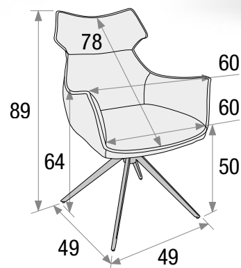
articolo 2342 Poltrona girevole struttura metallo rivestita in tessuto bianco e nero. imballo 1 pz. colli 1 - m 3 cartone 0,20 cm. l. 64,5 p. 60 h. 89 h.s. 50
