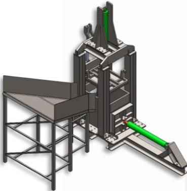
Diseño de prensa vertical de rebabeo metálico.
