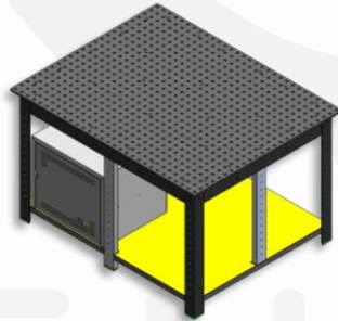
Diseño de mesa perforada para soldadura.
