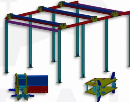
Diseño de estructura para transporte de carga.
