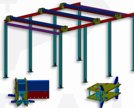
Diseño de estructura para transporte de carga.
