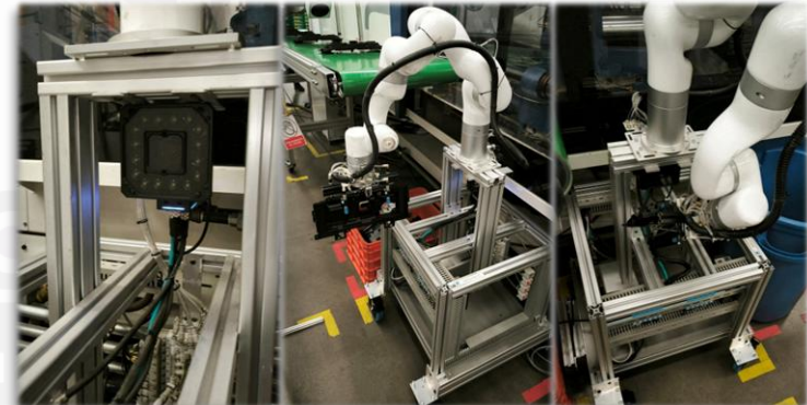
Programación e instalación cobot UFactory y cámara de visión.
