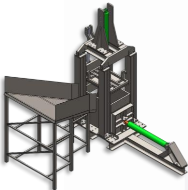
Diseño de prensa vertical de rebabeo metálico.
