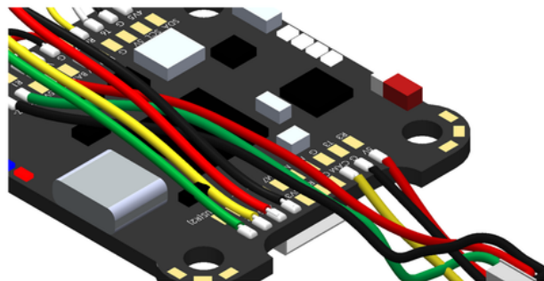
Teisingas laidų prilitavimas prie Skrydžio Valdiklio (FC)
