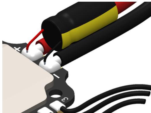
Maitinimo laidų (48) prilitavimas prie Greičio Regulatoriaus (14)
