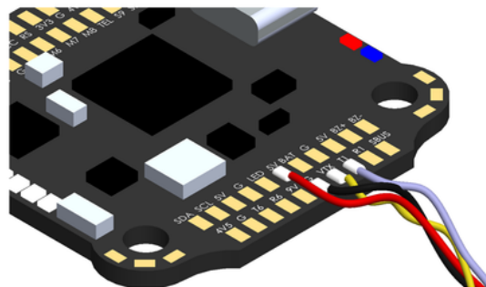
Teisingas laidų prilitavimas prie Skrydžio Valdiklio (FC)
