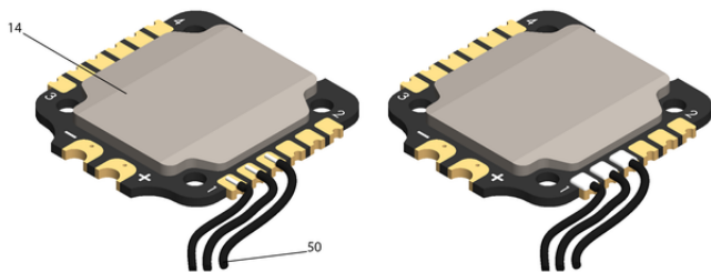
1-ojo variklio laidų litavimas
