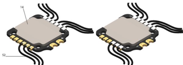
3-iojo variklio laidų litavimas
