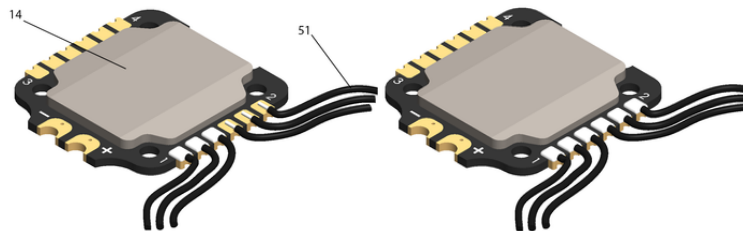
2-ojo variklio laidų litavimas
