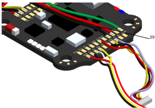
Pridėkite laidus prie atitinkamų padų.
