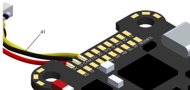
Pridėkite laidus prie atitinkamų padų.
