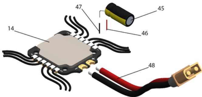
Kondensatorius (45) ir Maitinimo laidai (48) Greičio Reguliatoriui (14)
