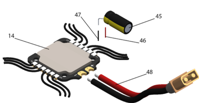
Kondensatorius (45) ir Maitinimo laidai (48) Greičio Reguliatoriui (14)
