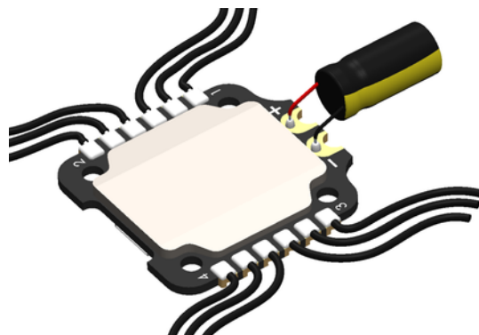
Kondensatoriaus (45) prilitavimas prie Greičio Reguliatoriaus (14)
