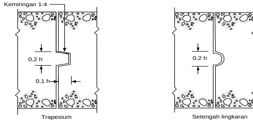
Gambar 5 Ukuran standar penguncian sambungan memanjang
