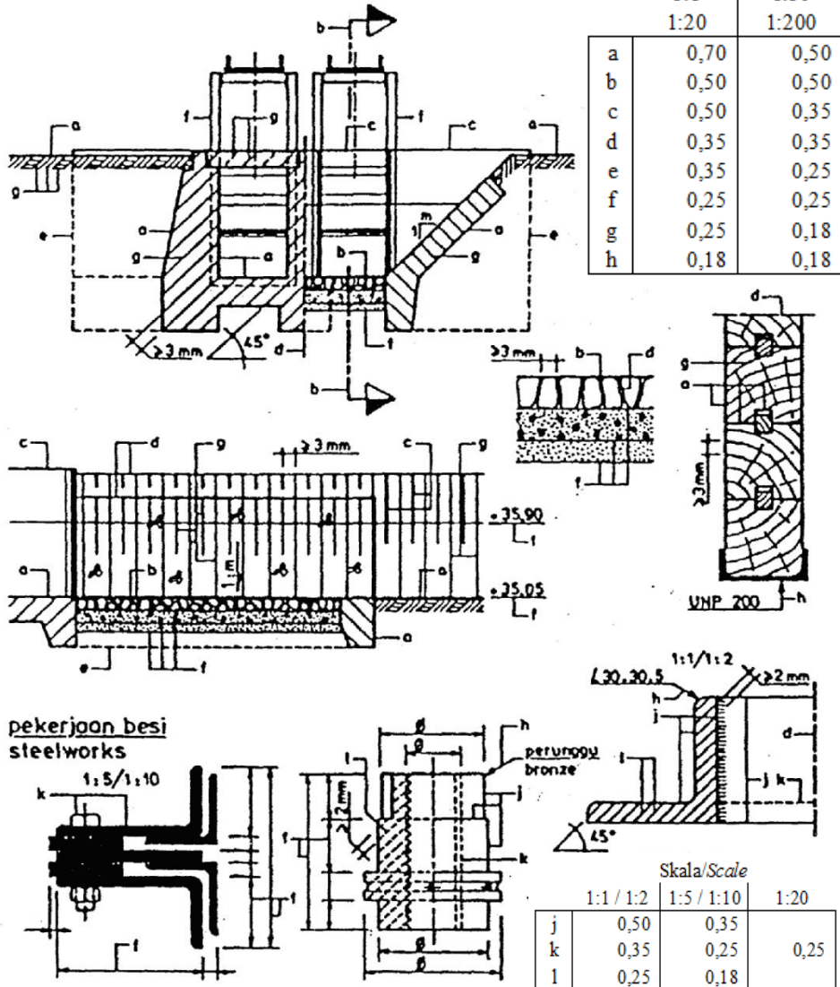
Gambar 7-1. Tebal Garis untuk Gambar-Gambar Bangunan
