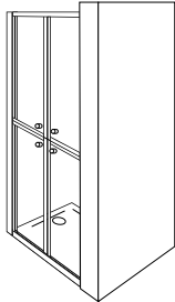
parete doccia con porta battente sdoppiata interno & esterno per installazione in nicchia
