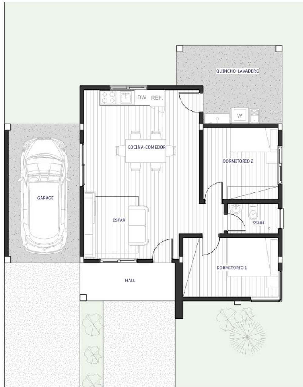
PLANTA EQUIPADA ESC. 1.50
