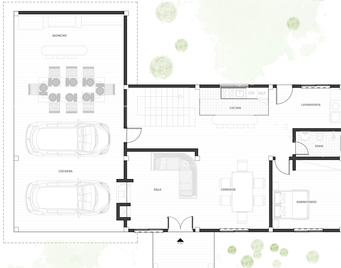
PLANTA NIVEL 1 EQUIPADA ESC. 1:100
