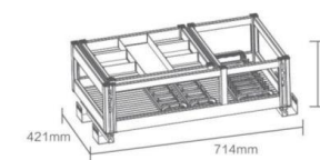
· 明星全铝三七抽（二合一）（上层） · KL750-37MC / 750柜体
