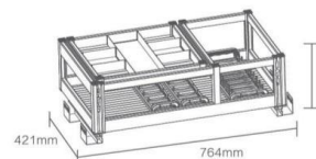
· 明星全铝三七抽（二合一）（上层） · KL800-37MC / 800柜体
