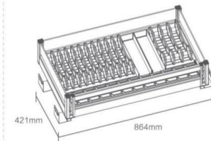
· 明星二合一通用碗盘抽 · KL900-MX4 / 900柜体
