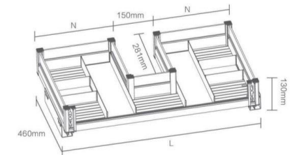
· 卫浴收纳篮 · DZ-WY46
