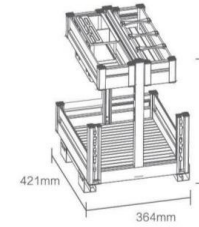
· 明星调味篮 · KL400-MX / 400柜体
