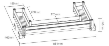
· 定制水槽收纳盖-大U (二合一) · KL01-SD34-900 / 900柜体
