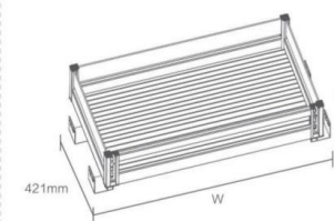
· 明星二合一通用碗盘抽(平抽) · 600-900柜体
