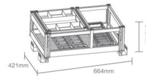
· 明星全铝三七抽（二合一）（上层） · KL700-37MC / 700柜体
