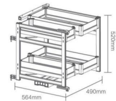
· 全铝地柜联动篮 · KL60-500 / 600柜体
