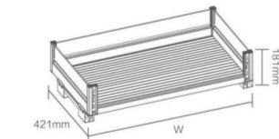
· 明星平篮 · 600-900柜体
