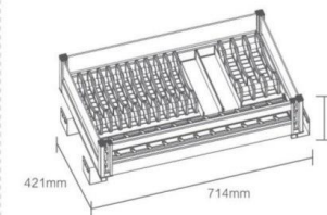
· 明星二合一通用碗盘抽 · KL750-MX4 / 750柜体
