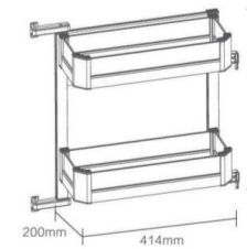
· 侧开连动百纳宝-2层 · KL45-C / 450柜体
