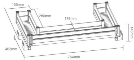
· 定制水槽收纳盖-大U (二合一) · KL01-SD34-800 / 800柜体
