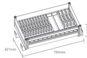
· 明星二合一通用碗盘抽 · KL800-MX4 / 800柜体
