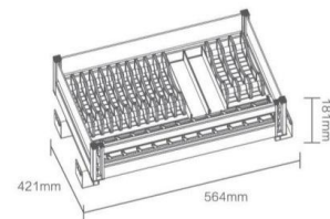
· 明星二合一通用碗盘抽 · KL600-MX4 / 600柜体
