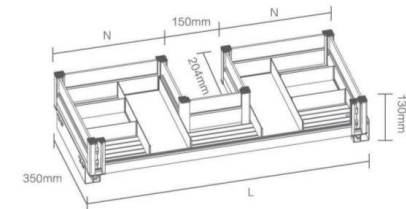
· 卫浴收纳篮 · DZ-WY35
