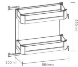
· 侧开连动百纳宝-2层 · KL60-C / 600柜体
