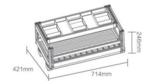
· 明星碗盘抽中抽 · KL750-MC / 750柜体
