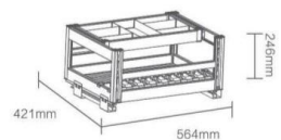
· 明星碗盘抽中抽 · KL600-MC / 600柜体
