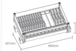
· 明星二合一通用碗盘抽 · KL700-MX4 / 700柜体
