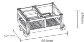
· 明星全铝三七抽（二合一）（上层） · KL600-37MC / 600柜体
