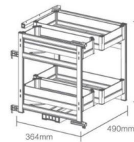
· 全铝地柜联动篮 · KL40-500 / 400柜体
