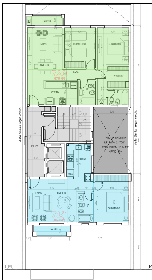
FRENTE planta 7º piso
