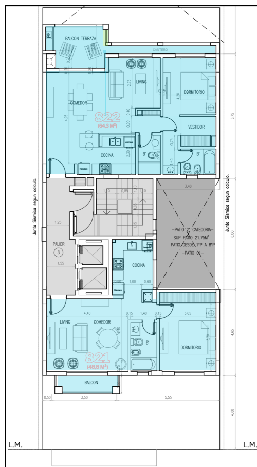
FRENTE planta 8º piso
