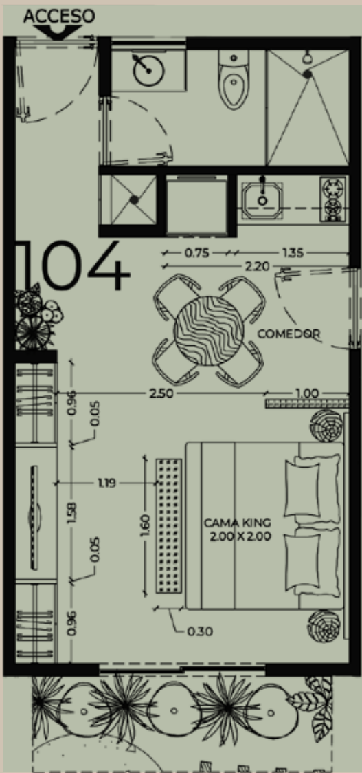
ESTUDIO TIPO B STUDIO TYPE B
