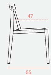
Solid Silla Madera de haya. Asiento acolchado y tapizado. Beech wood. Padded and upholstered seat.
