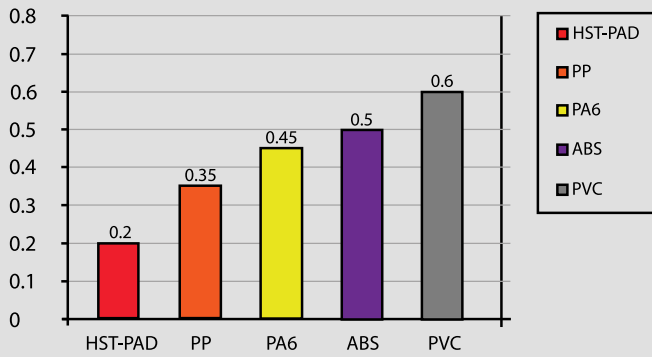
마찰 계수
