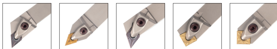
DDJN□93° DDPNN62.5° DDQN□107.5° DSBN□75° DSDNN45°
