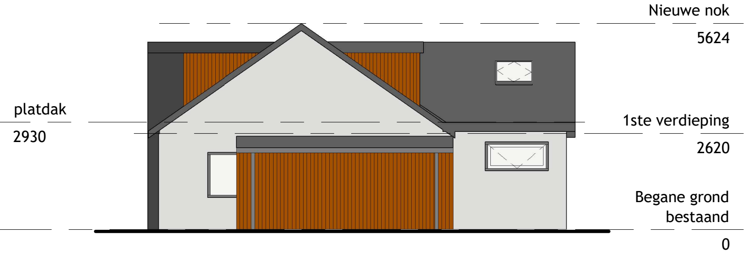
Voorgevel nieuw
