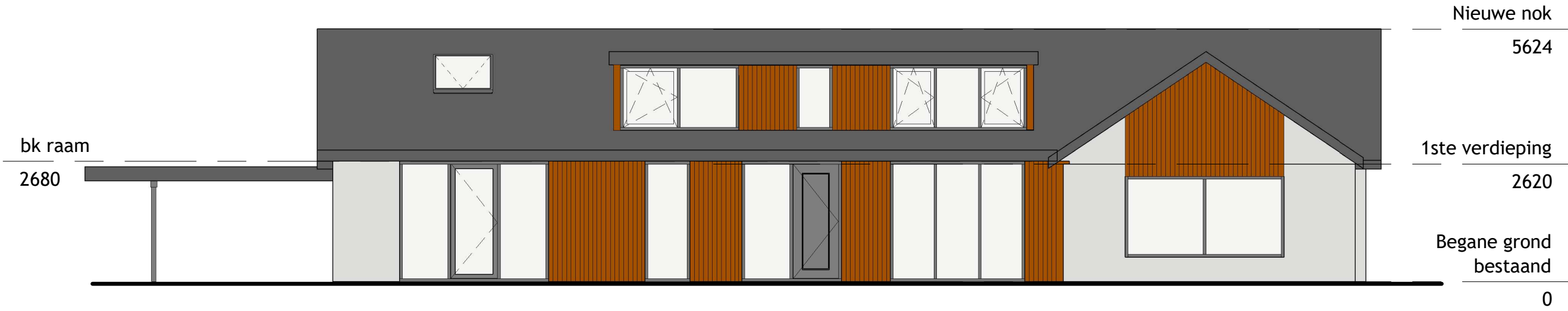
Rechtergevel nieuw
