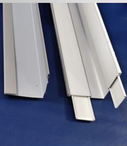
الزاوية الخارجية وخفي المسمار والزاوية القياسية الالواح ٣متر
