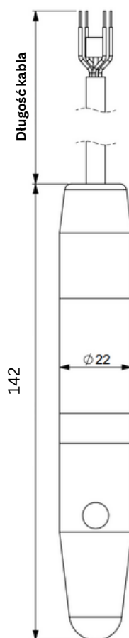
Sonda z obciążnikiem stalowym lub z tworzywa
