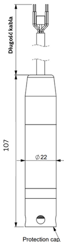
Sonda z osłoną ochronną z tworzywa sztucznego
