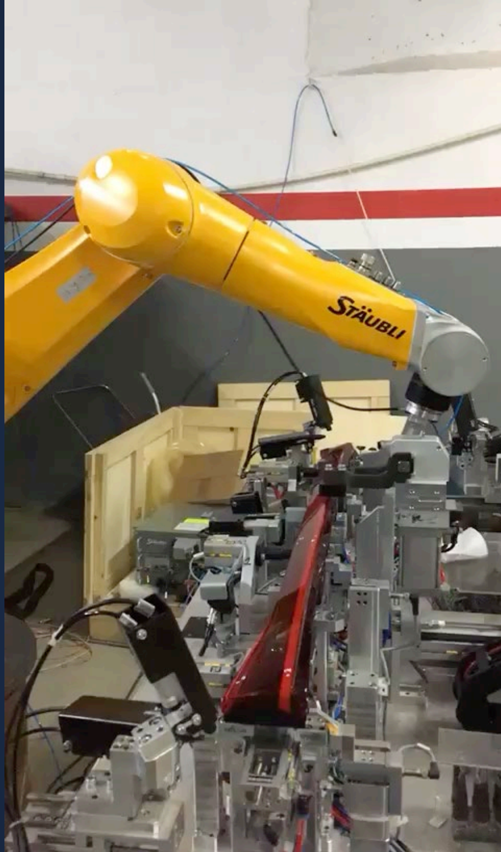
Arka Far Boyutsal Ölçüm Makinesi
