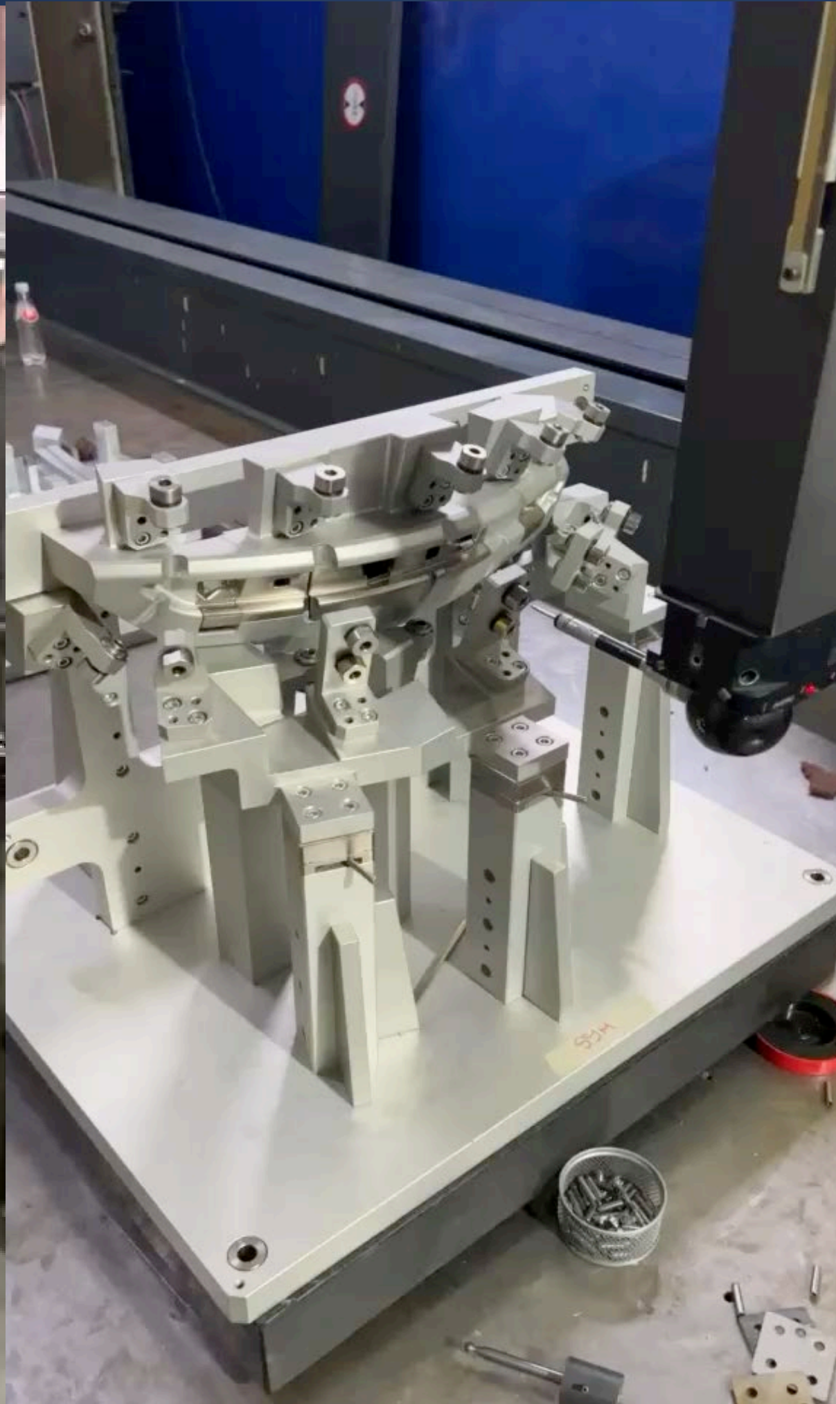
CMM Ölçüm Fikstürü
