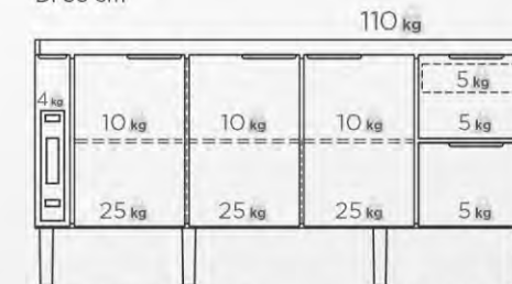
CABINET W: 174 / 194 cm H: 85 cm D: 51 cm
