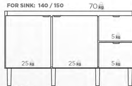
CABINET W: 134 / 144 cm H: 78,7 cm D: 51 cm
