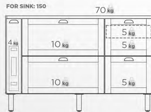
CABINET W: 144,1 cm H: 91 cm D: 51,5 cm
