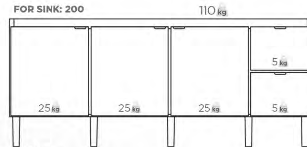
CABINET W: 194 cm H: 78,7 cm D: 51 cm
