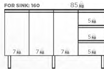
CABINET W: 153,6 cm H: 84,8 cm D: 49,8 cm
