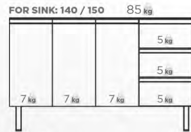
CABINET W: 134,7 / 144,5 cm H: 84,8 cm D: 49,8 cm
