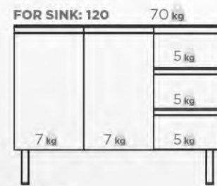
CABINET W: 117 cm H: 84,8 cm D: 49,8 cm
