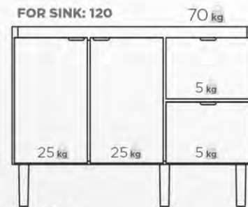
CABINET W: 114 cm H: 78,7 cm D: 51 cm
