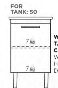
WASHING TANK CABINET W: 49,5 cm H: 52 cm D: 42,1 cm
