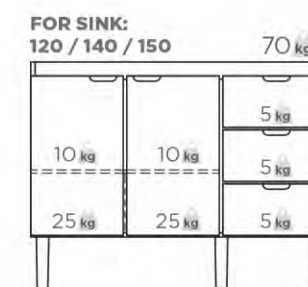
CABINET W: 114 / 134 / 144 cm H: 85 cm D: 51,1 cm
