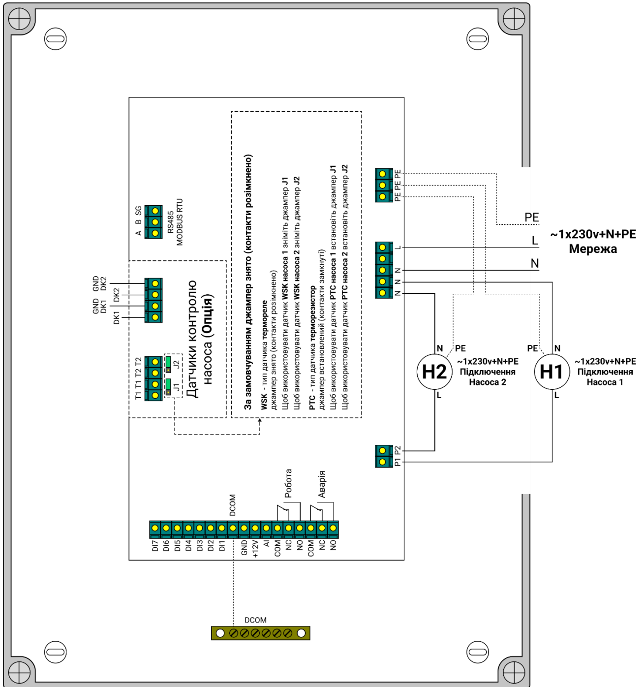
Мал 6 - Силові ланцюги приладу та насосів для моделей з прямим пуском.
