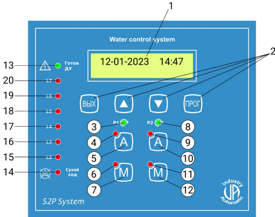
Мал 3 - Зовнішній вигляд панель керування. (для режиму “Підвищення тиску”)
