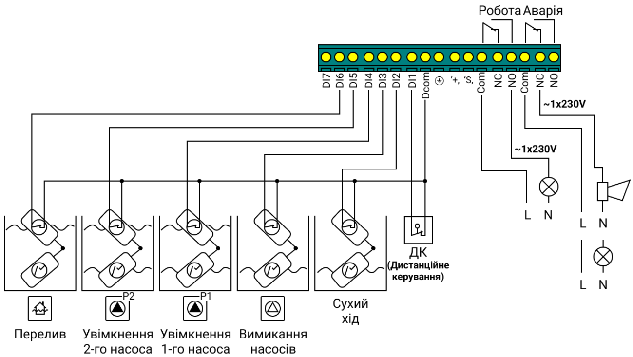
Мал 8 – Клемна колодка зовнішніх підключень сигнальних ланцюгів приладу у режимі «Відведення стоків». Поплавкові датчики.
