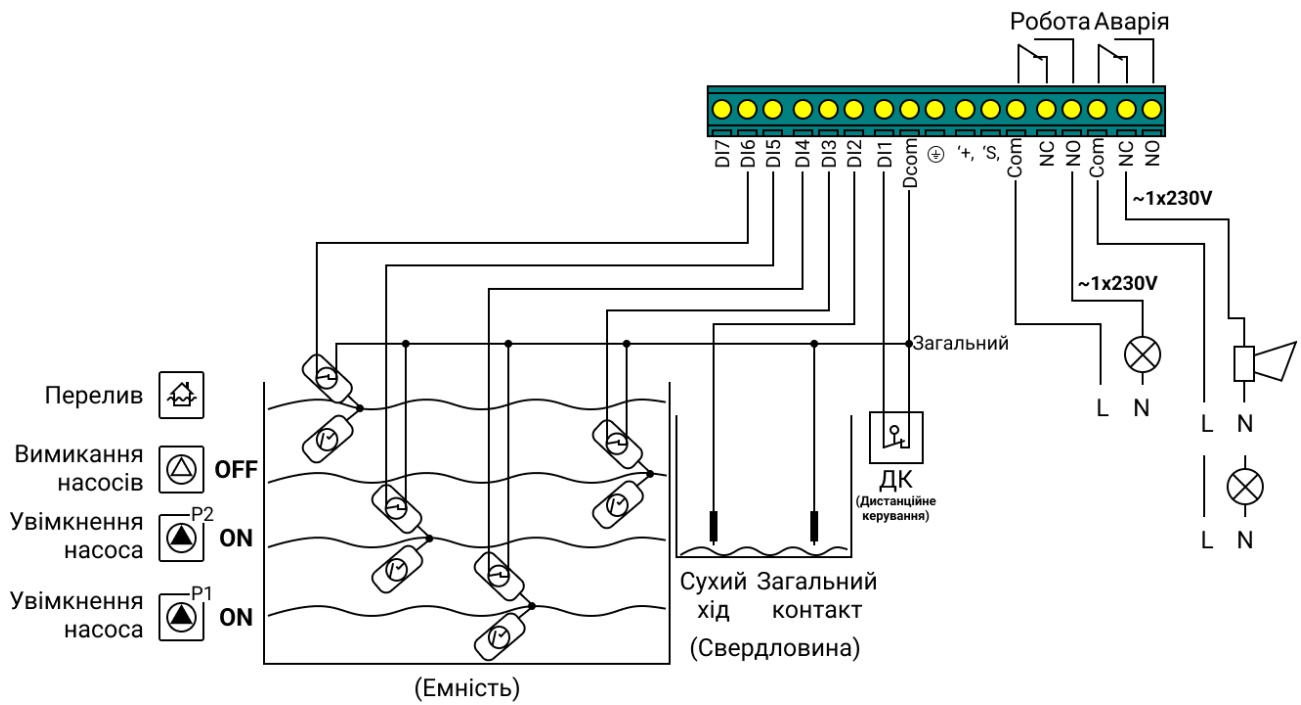
Мал 12 – Клемна колодка зовнішніх підключень сигнальних ланцюгів приладу у режимі «Наповнення».
