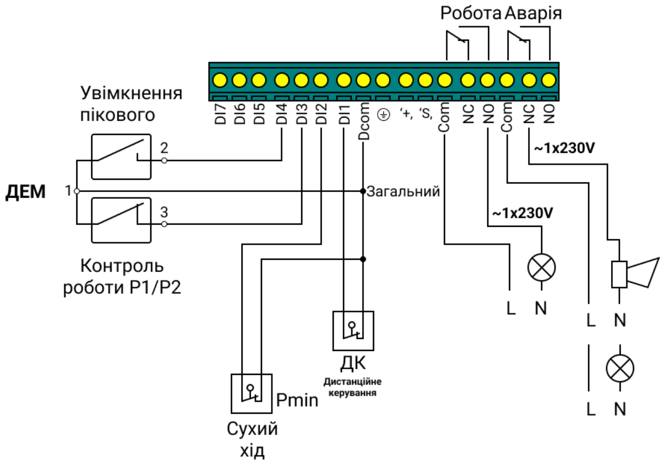
Мал 17 – Клемна колодка зовнішніх підключень сигнальних ланцюгів приладу у режимі «Циркуляція» . Диференціальний електроманометр, термостат пікового насосу, реле сухого ходу.
