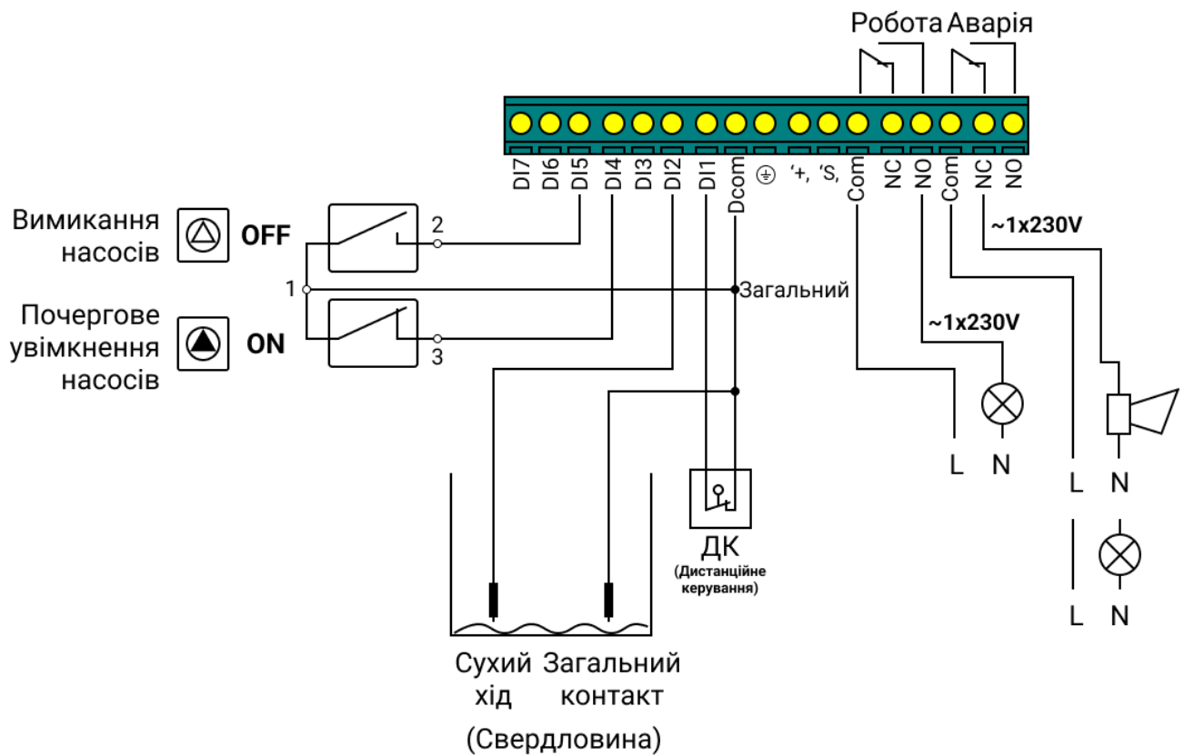
Мал 15 – Клемна колодка зовнішніх підключень сигнальних ланцюгів приладу у режимі «Підвищення тиску». Електроконтактний манометр типу V та електродні датчики.
