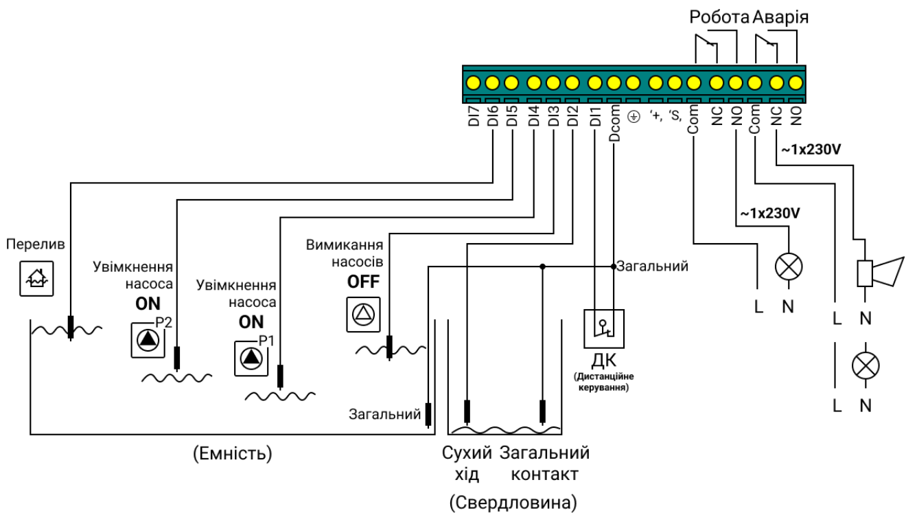
Мал 10 – Клемна колодка зовнішніх підключень сигнальних ланцюгів приладу у режимі «Наповнення».
