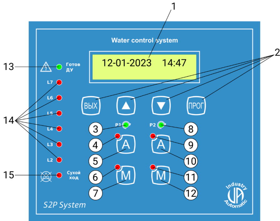
Мал 4 - Зовнішній вигляд панель керування. (для режиму “Циркуляція”)
