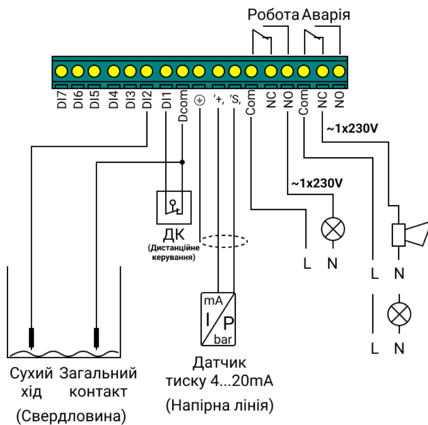
Мал 14 – Клемна колодка зовнішніх підключень сигнальних ланцюгів приладу у режимі «Підвищення тиску».
