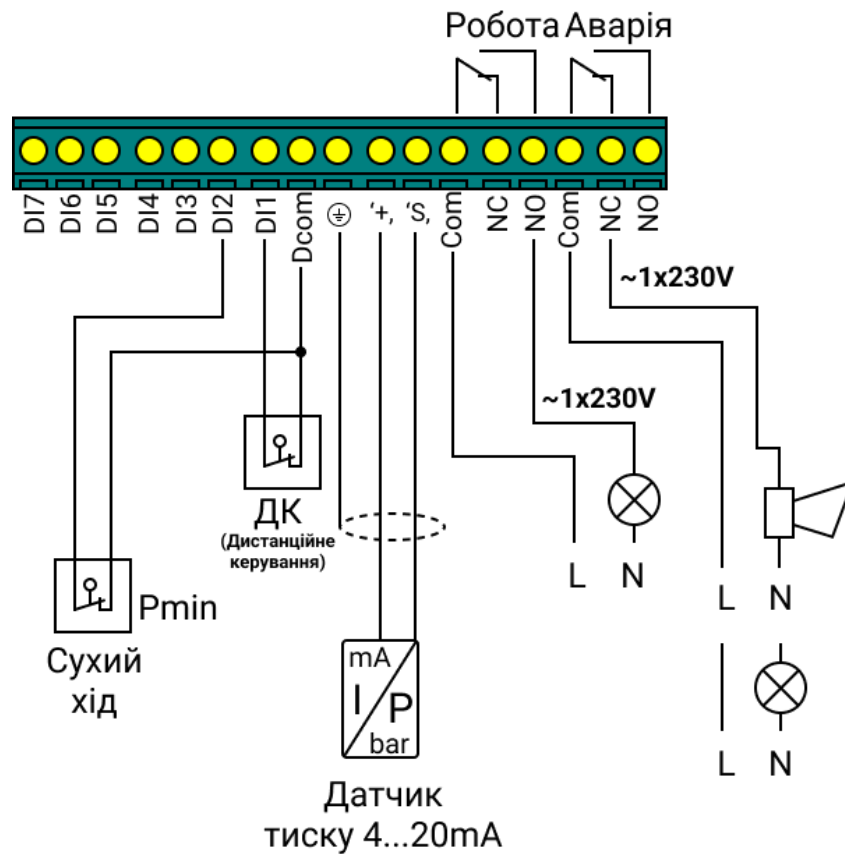
Мал 13 – Клемна колодка зовнішніх підключень сигнальних ланцюгів приладу у режимі «Підвищення тиску».
