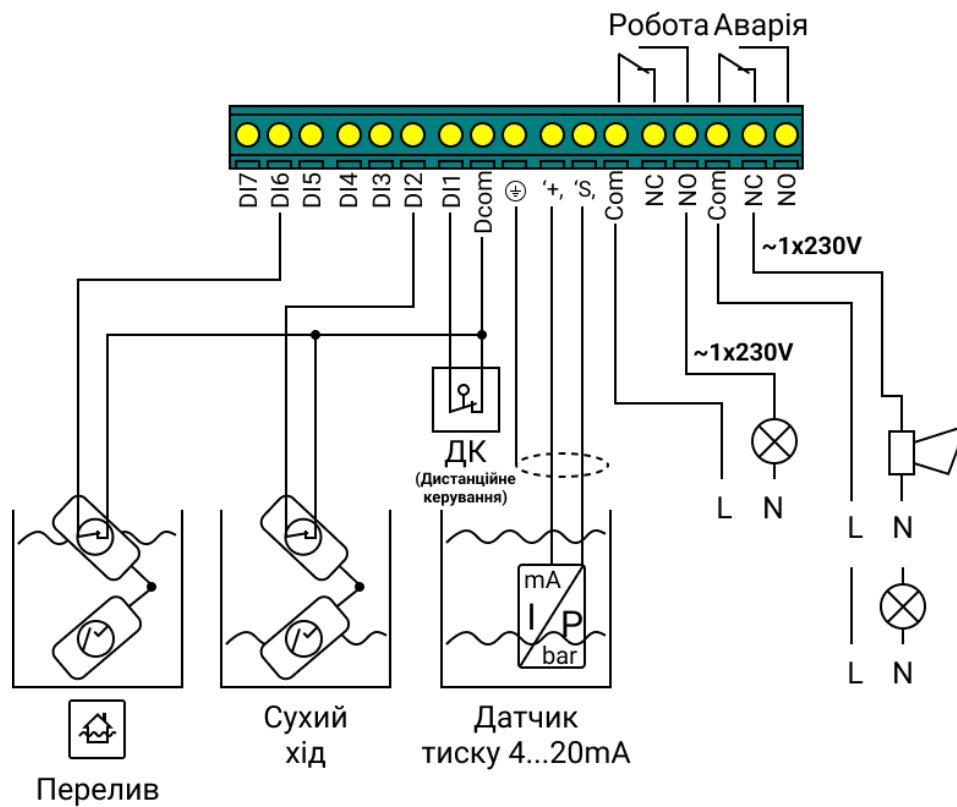
Мал 7 – Клемна колодка зовнішніх підключень сигнальних ланцюгів приладу у режимі «Відведення стоків». Датчик тиску 4–20мА та Поплавкові датчики.
