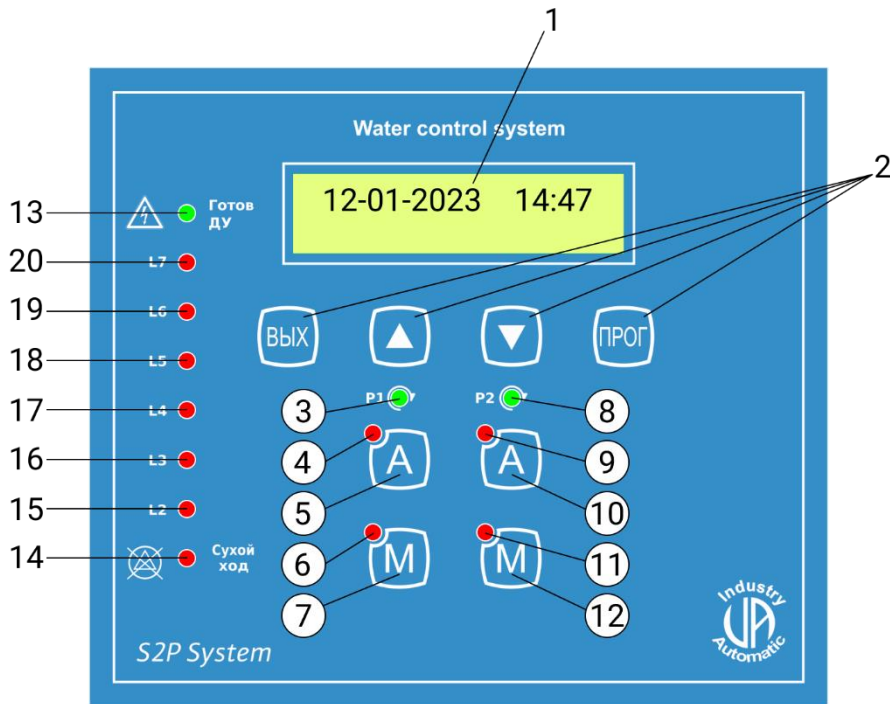
Мал 2 - Зовнішній вигляд панель керування. (для режиму “Наповнення”)
