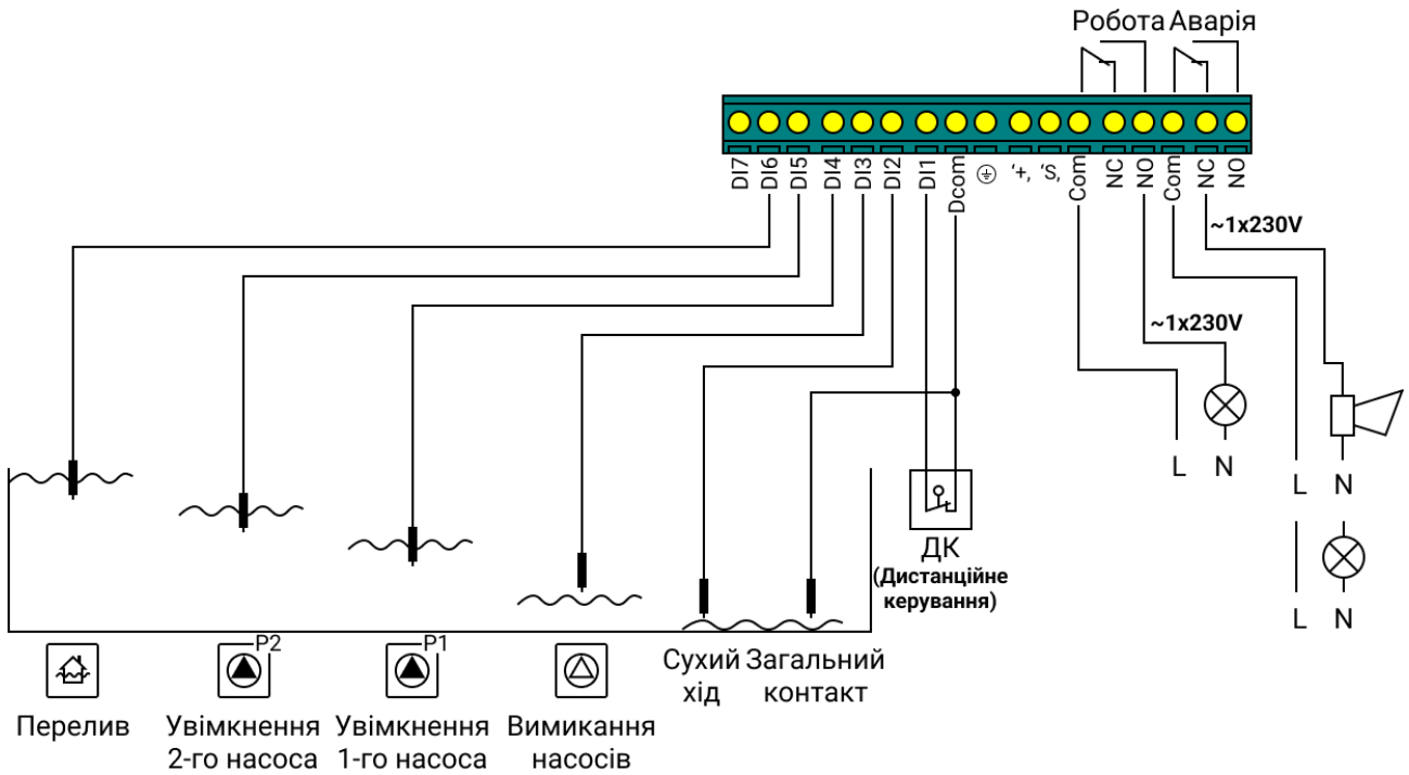
Мал 9 – Клемна колодка зовнішніх підключень сигнальних ланцюгів приладу у режимі «Відведення стоків». Електродні датчики.
