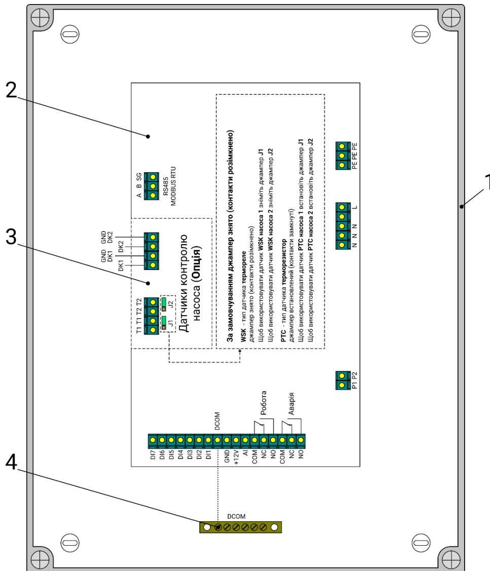
Мал 5 - Внутрішній вигляд приладу керування із прямим пуском насосів.
