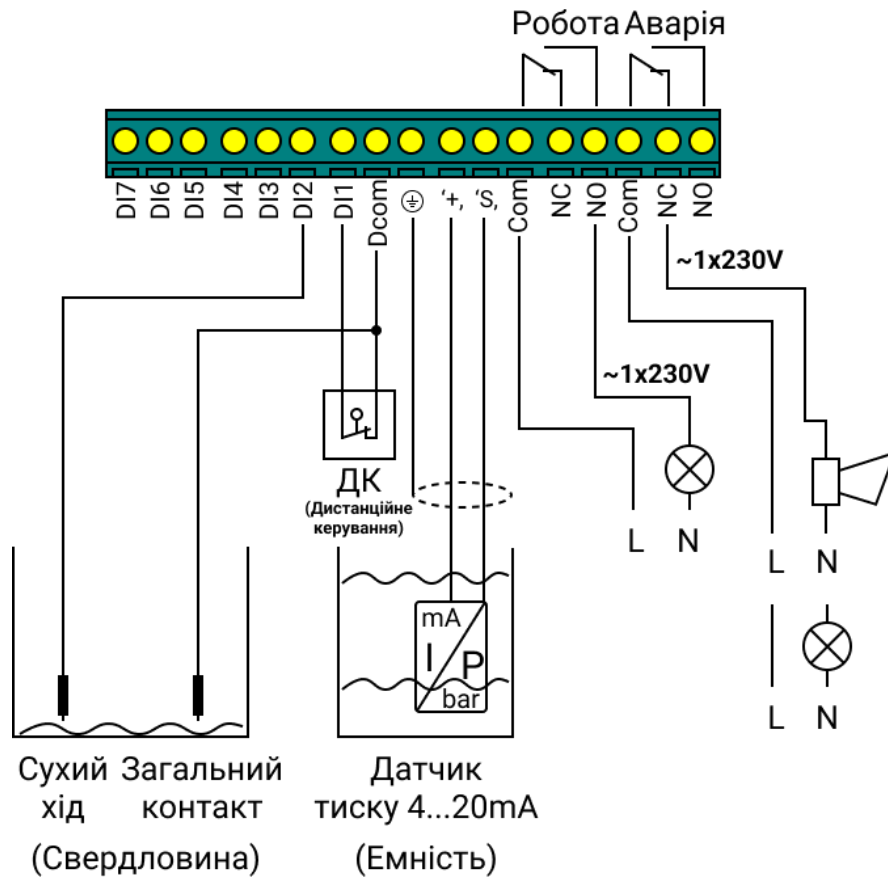
Мал 11 – Клемна колодка зовнішніх підключень сигнальних ланцюгів приладу у режимі «Наповнення».
