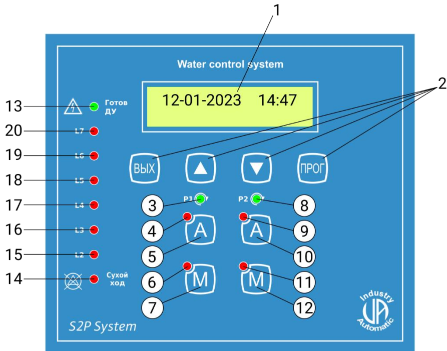
Мал 1 - Зовнішній вигляд панель керування. (для режиму “Відведення стоків”)
