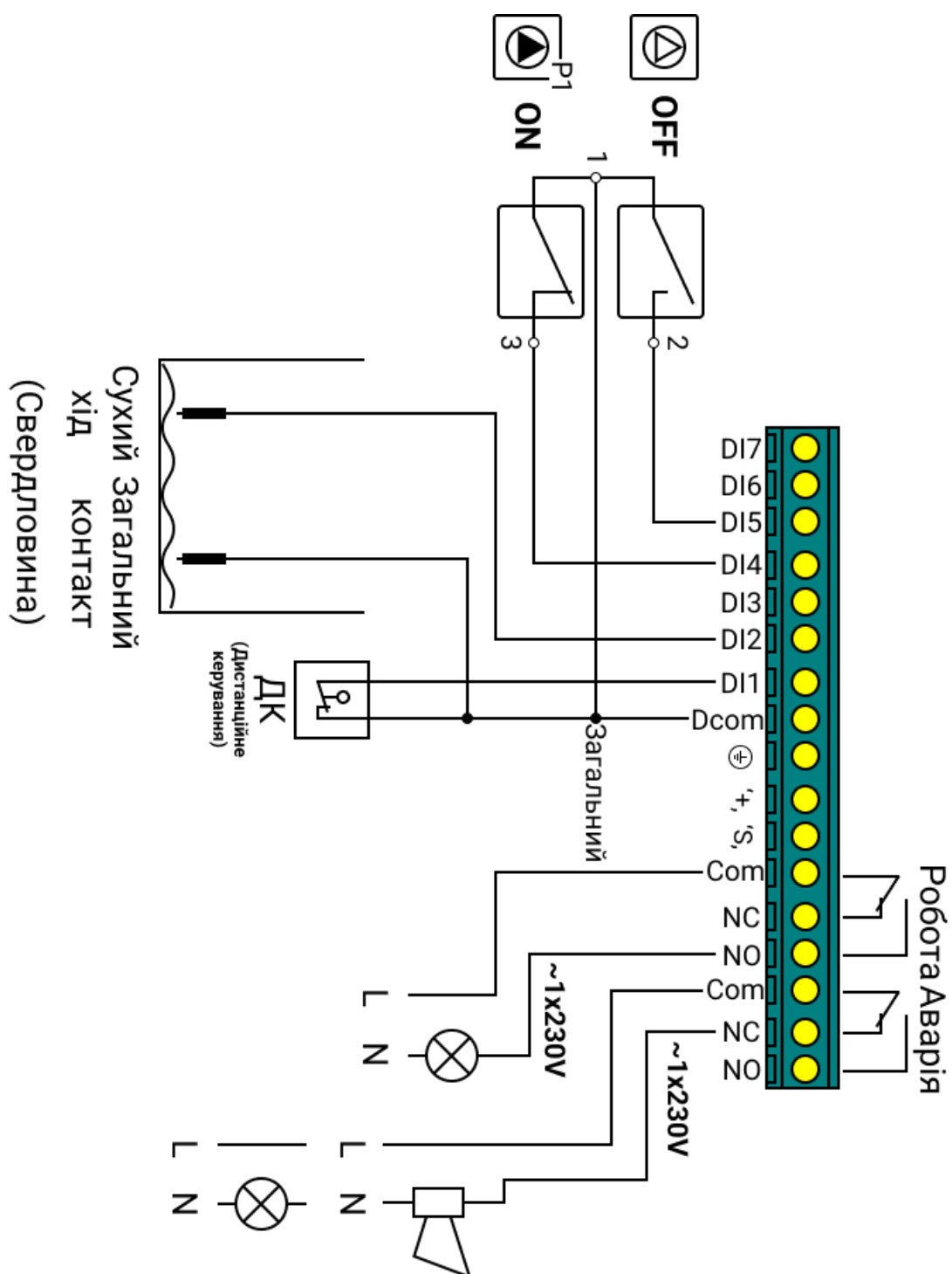
Мал 15 – Клемна колодка зовнішніх підключень сигнальних ланцюгів приладу у режимі «Підвищення тиску». Електроконтактний манометр типу V та електродні датчики.
