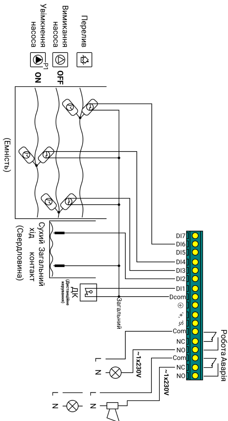
Мал 12 – Клемна колодка зовнішніх підключень сигнальних ланцюгів приладу у режимі «Наповнення». Поплашкові датчики та Електродні датчики.
