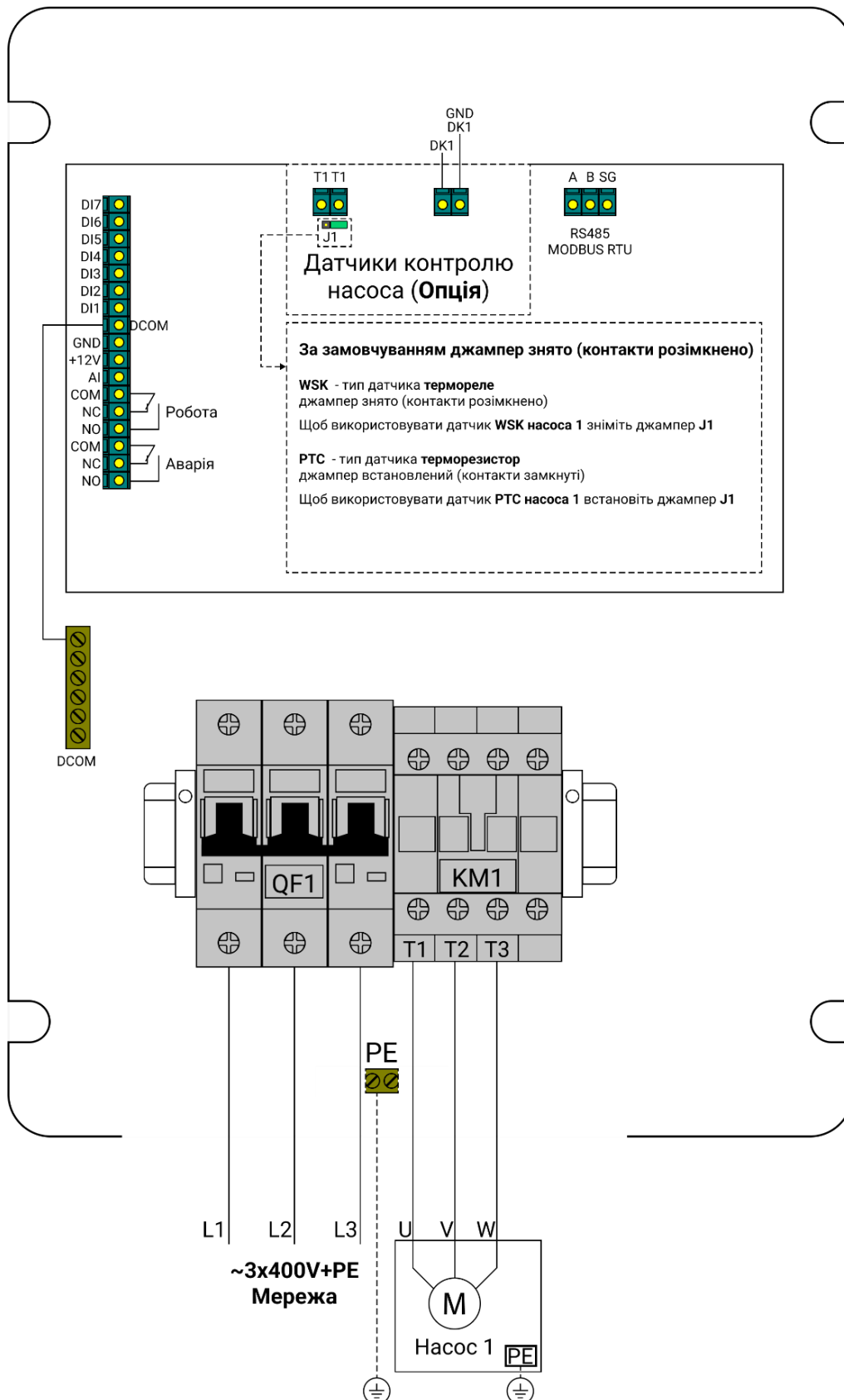
Мал 6 - Силові ланцюги приладу та насоса для моделей з прямим пуском.
