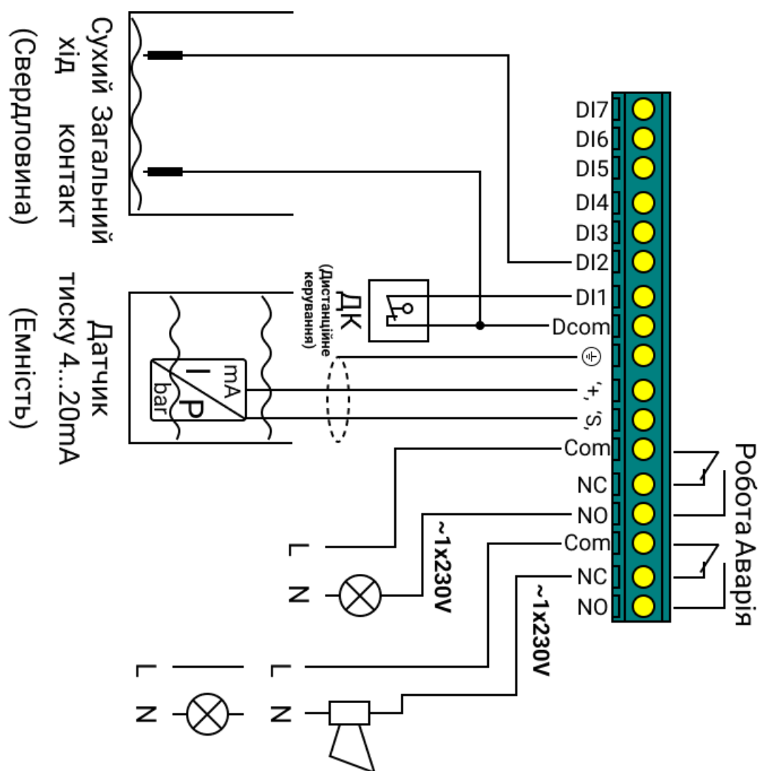
Мал 11 – Клемна колодка зовнішніх підключень сигнальних ланцюгів приладу у режимі «Наповнення». Датчик тиску 4–20mA та Електродні датчик.
