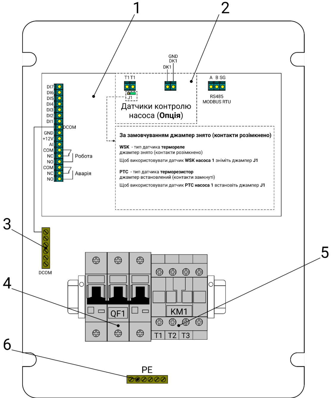
Мал 5 - Внутрішній вигляд приладу керування із прямим пуском насоса.
