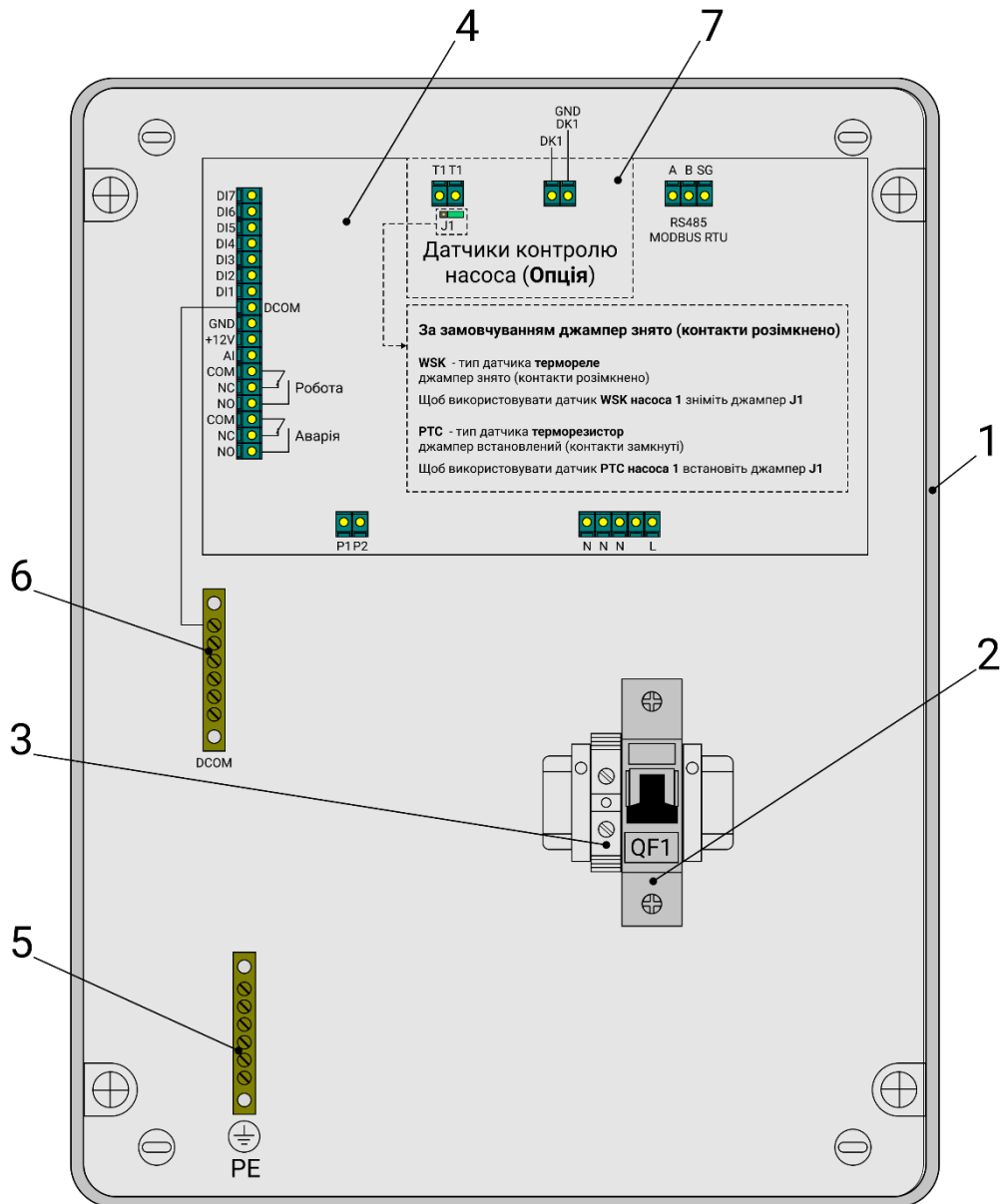
Мал 5 - Внутрішній вигляд приладу керування з прямим пуском насоса.
