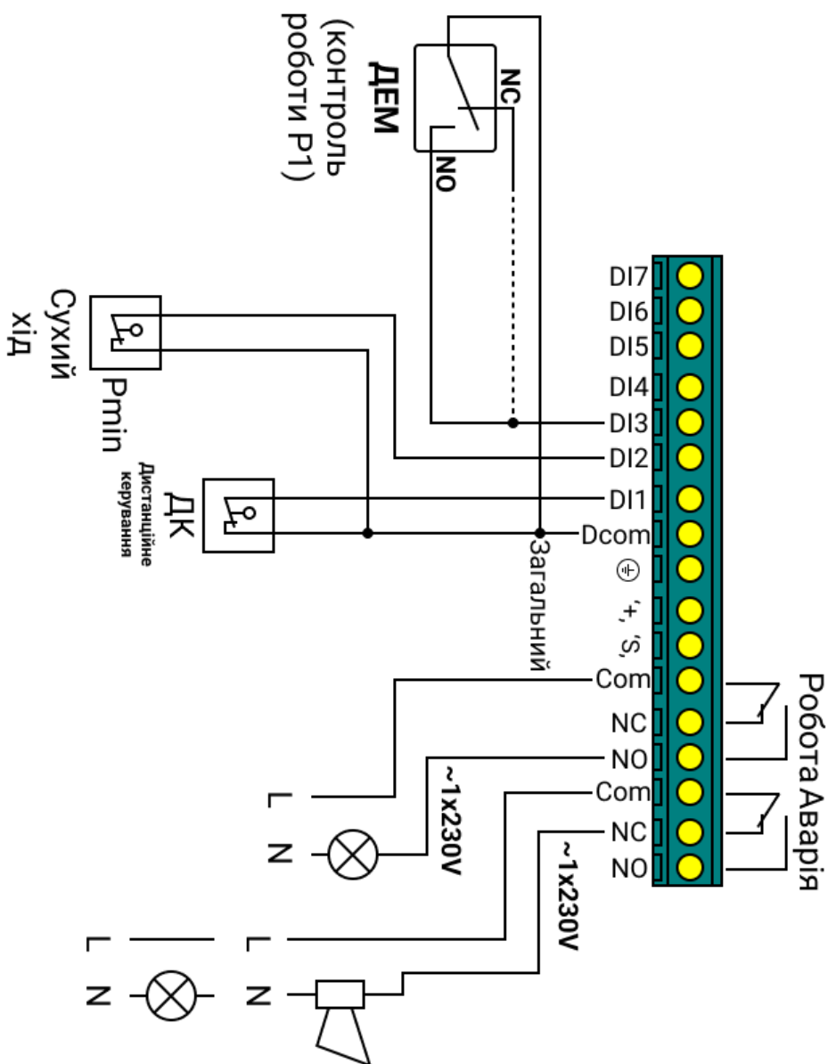
Мал 17 – Клемна колодка зовнішніх підключень сигнальних ланцюгів приладу у режимі «Циркуляція». Диференціальний електроманометр та реле сухого ходу.
