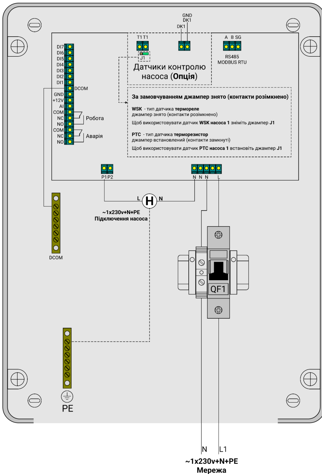
Мал 6 - Силові ланцюги приладу та насоса з прямим пуском.
