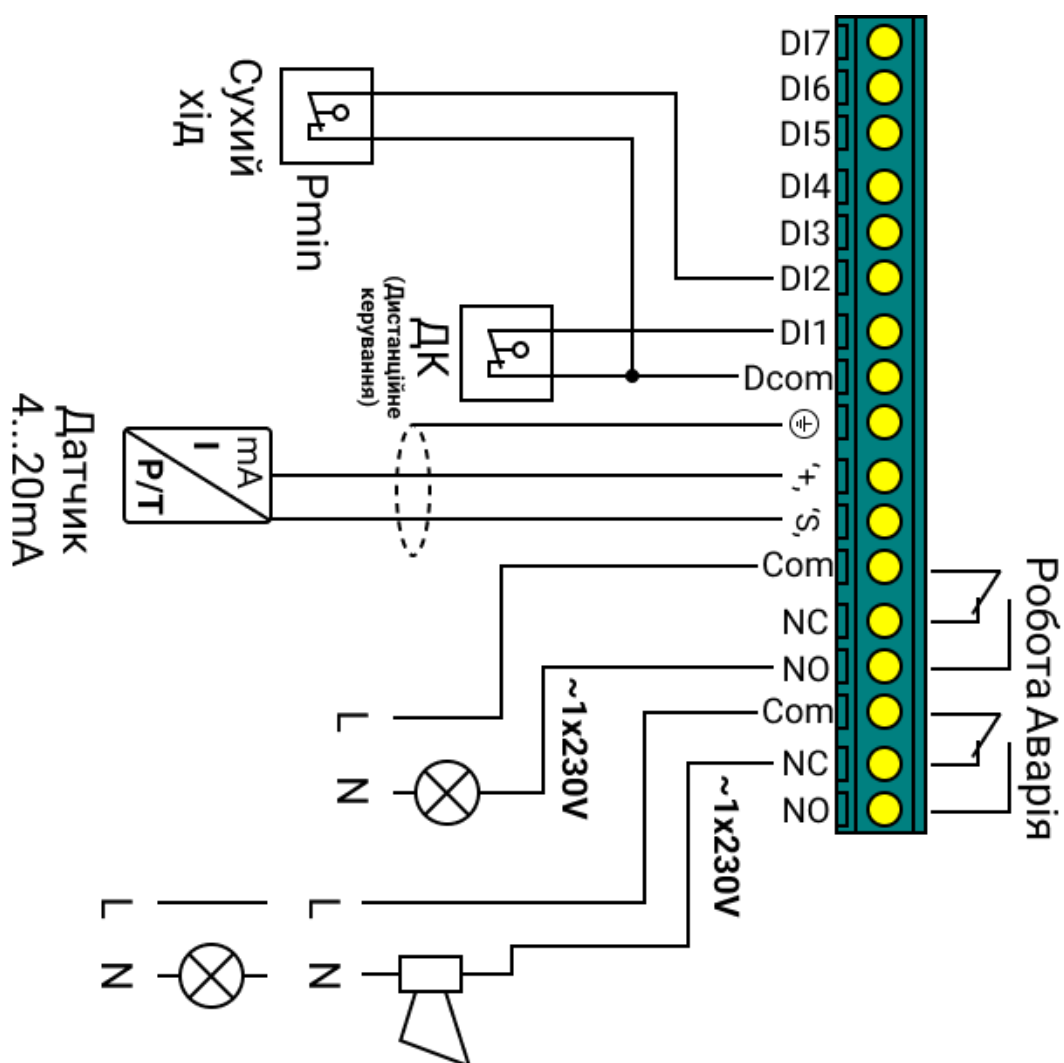
Мал 16 – Клемна колодка зовнішніх підключень сигнальних ланцюгів приладу у режимі «Циркуляція».
