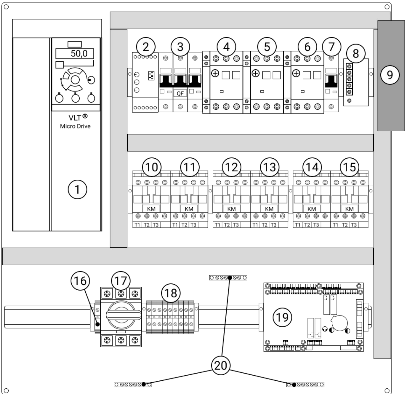
Конструктивні елементи приладу керування (Можливі зміни приладу, що не порушують функціональність)
