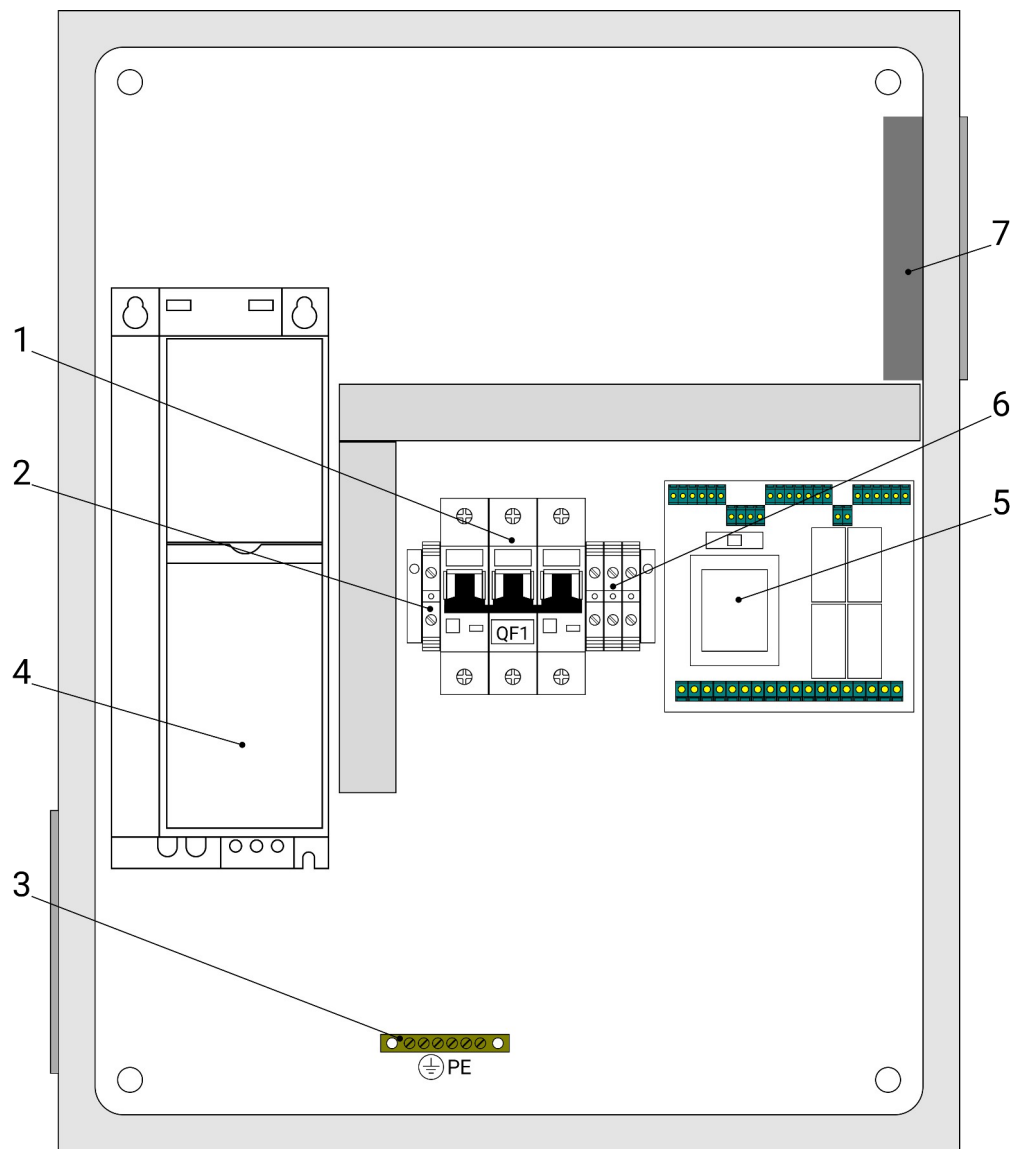
Мал.2. – Внутрішній вигляд приладу керування.
