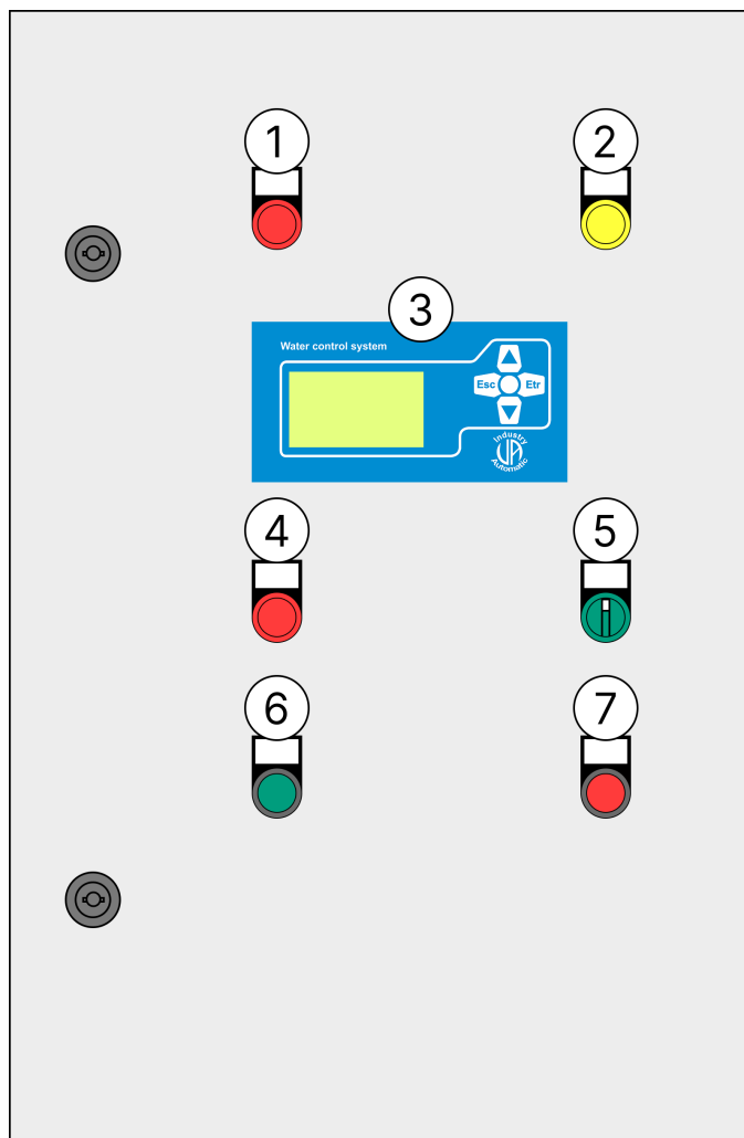
Мал.1 – Зовнішній вигляд
