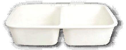
الموديل: ST2 العمق: 20.5 الوزن (كغ): 18 الطول: 71 العرض: 41
