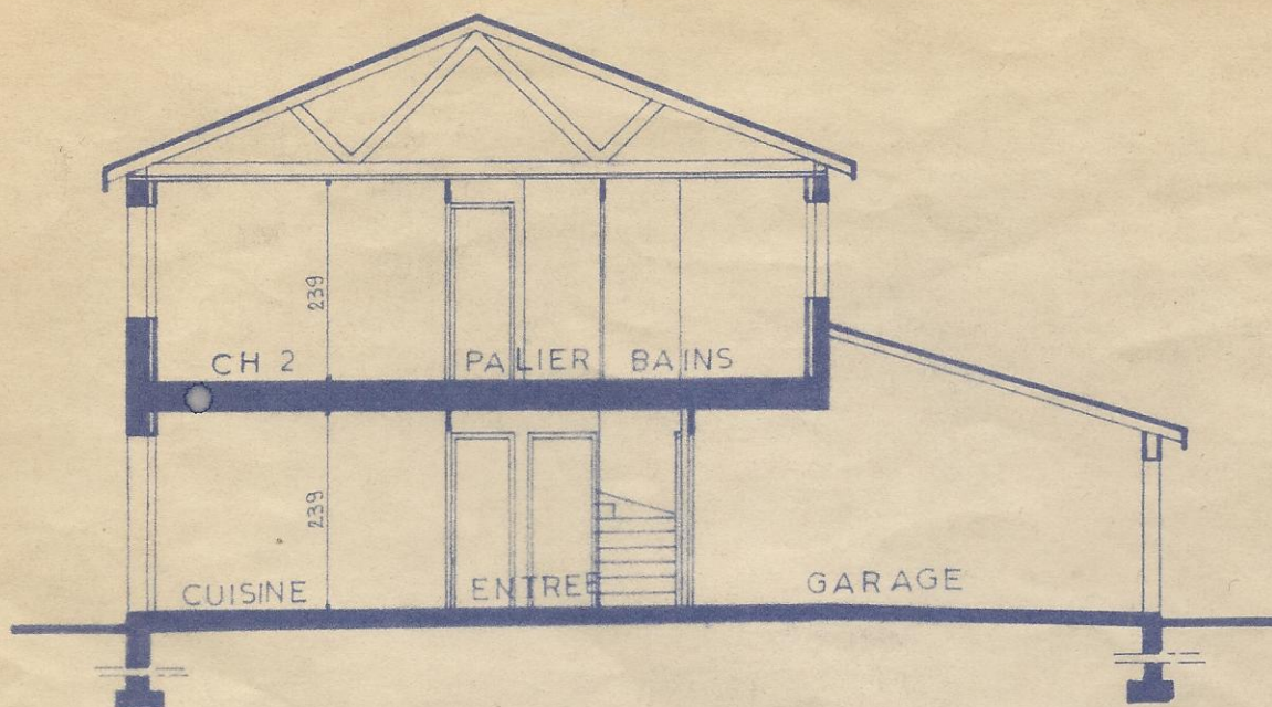
COUPE
