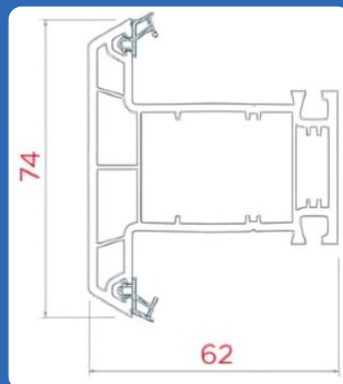
AST - 621 - TO1 T - MULLION
