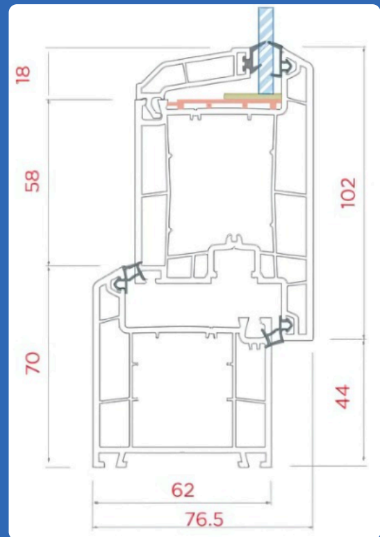
AST - 621 - TO2 Z - MULLION
