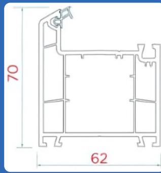
AST - 621 - FO2 DOOR OUTER FRAME
