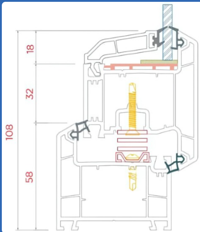
AST - 621 - SO4 INWARD OPENING DOOR SASH
