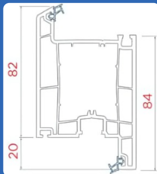
AST - 621 - SO4 INWARD OPENING DOOR SASH
