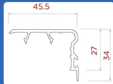
AST - 621 - L02 INTERLOCK FOR DOOR SASH
