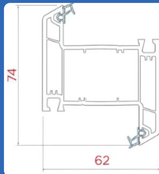
AST - 621 - TO2 Z - MULLION
