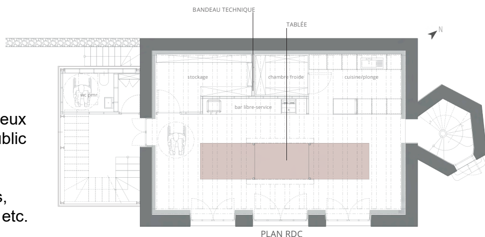
PLAN RDC
