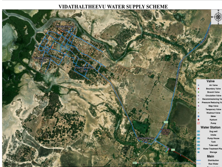
படம் 5விடத்தல்தீவு நீர் வழங்கல் திட்டத்தின் வரைபடம்
