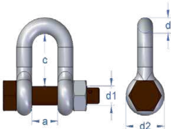
Grillete N° 835 con perno de seguridad.
