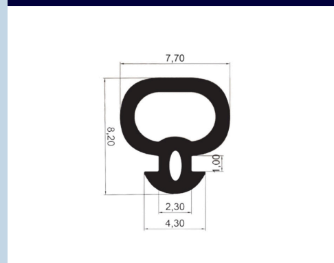
GAXETA DA COLUNA E TRAVESSA FAA 202/2 / TP 269
