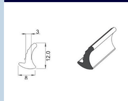
GUARNIÇÃO PARA VIDRO 10MM GUA 038N PRETA
