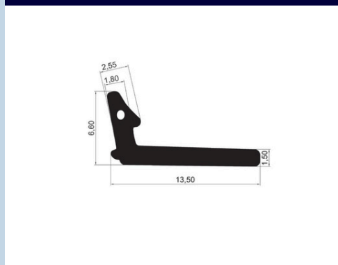
GAXETA EXTERNA FAA 250
