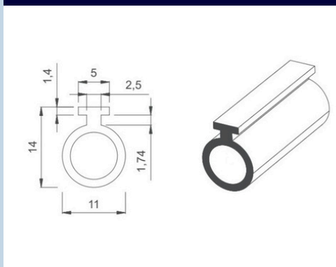
GUARNIÇÃO PARA PINGADEIRA SUPREMA GUA 007 PRETA
