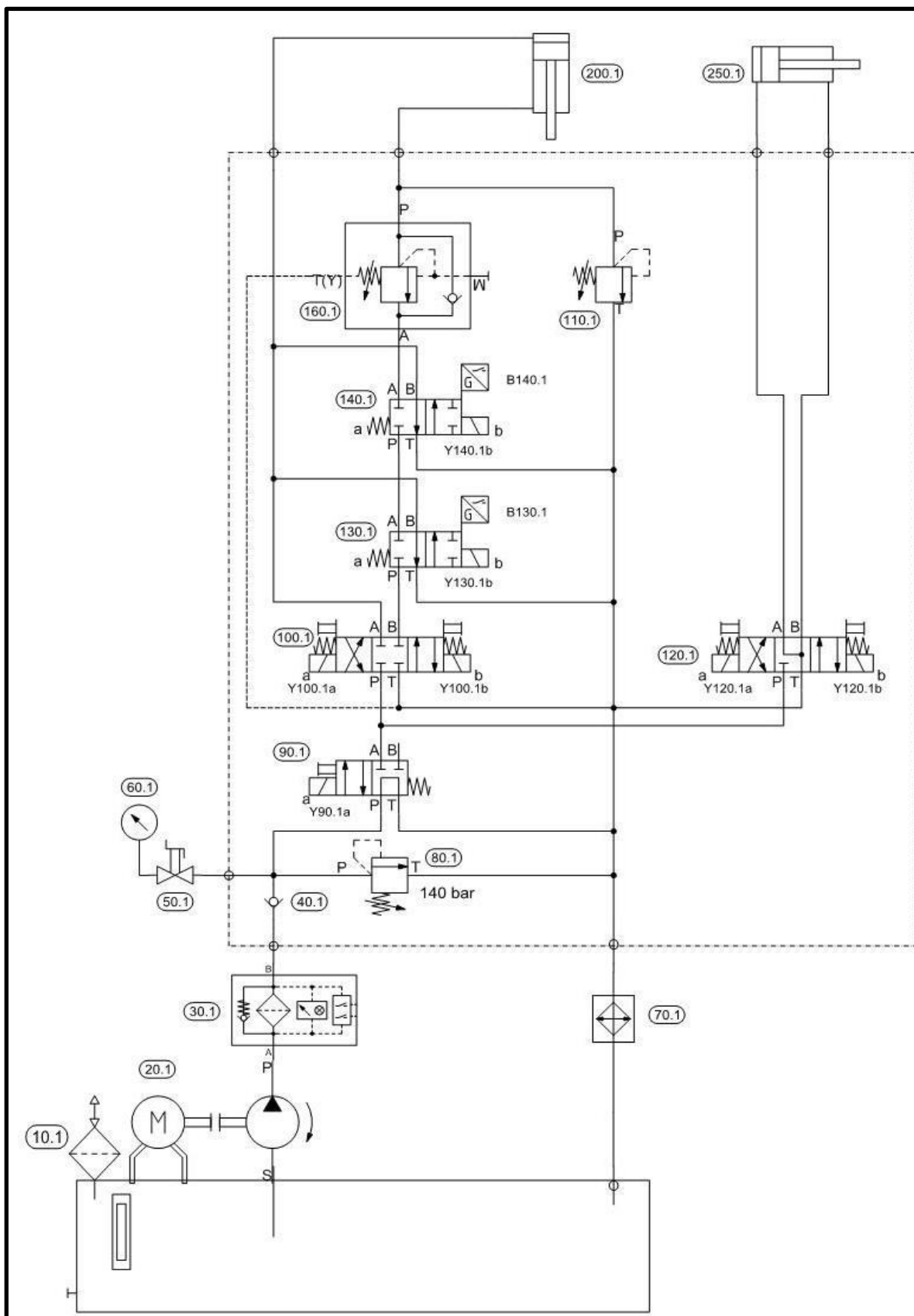
Figura 94: Circuito hidráulico
