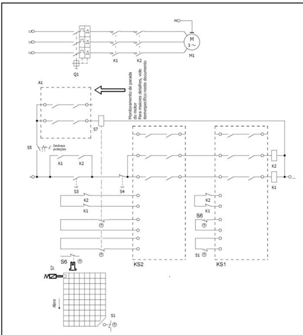
Figura 89: Circuito elétrico
