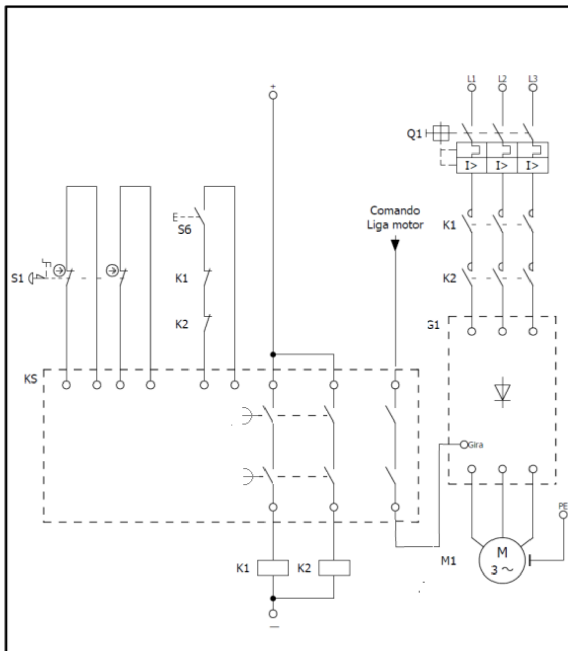
Figura 77: Circuito elétrico
