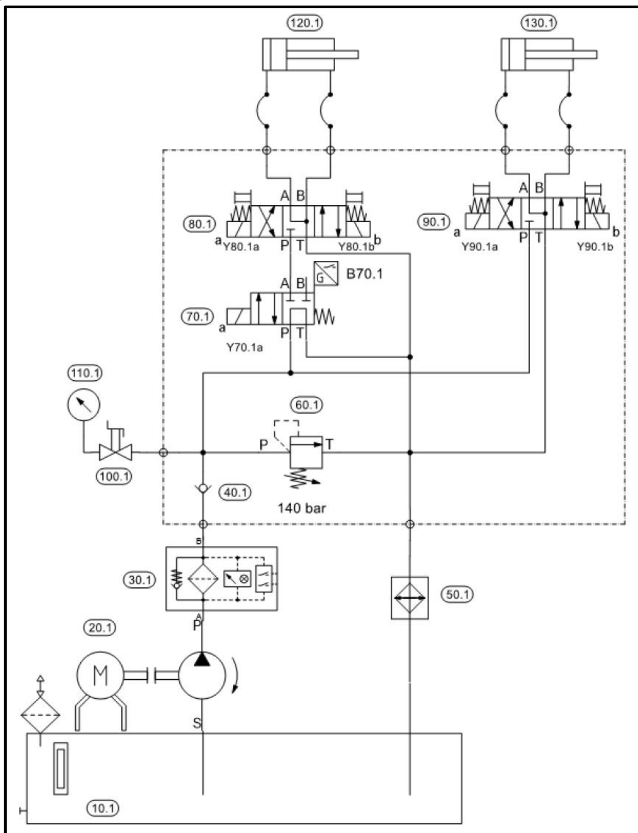
Figura 103: Circuito hidráulico
