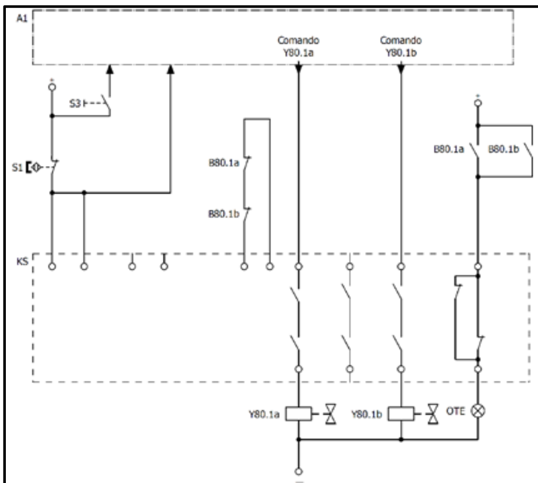
Figura 44: Circuito elétrico
