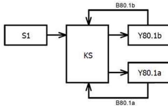
Figura 46: Representação de blocos - parada relacionada à segurança
