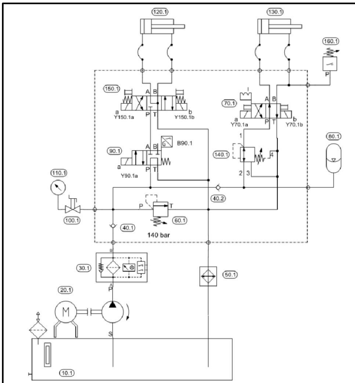
Figura 63: Circuito hidráulico
