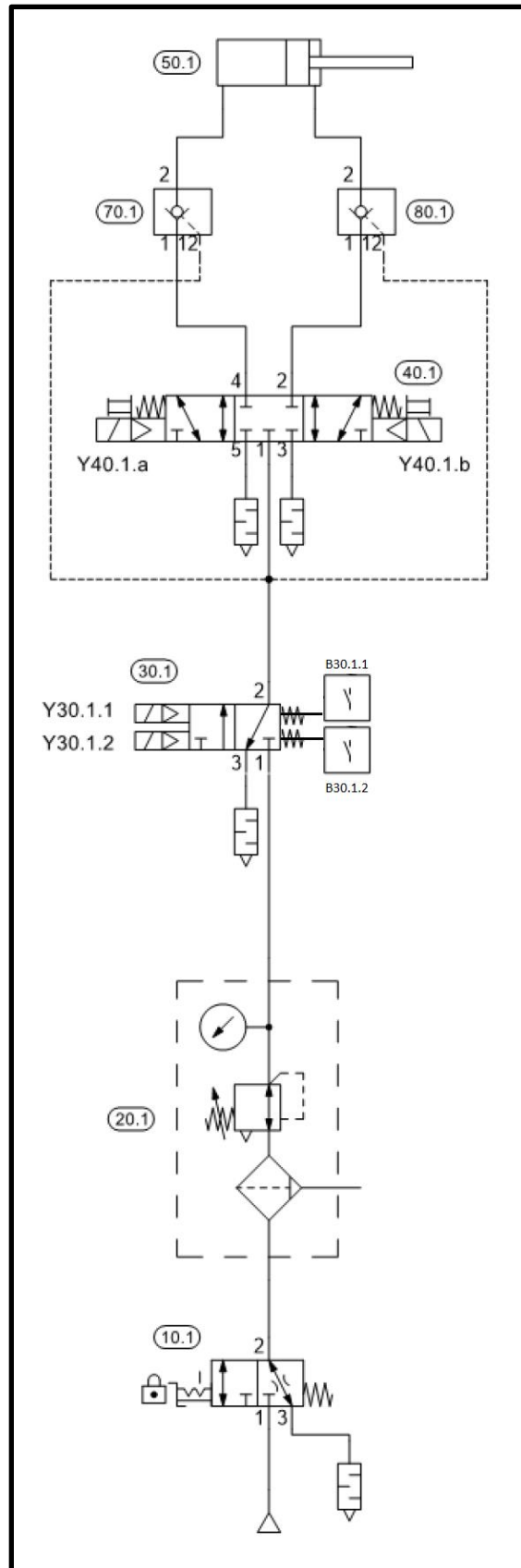
Figura 101: Circuito neumático
