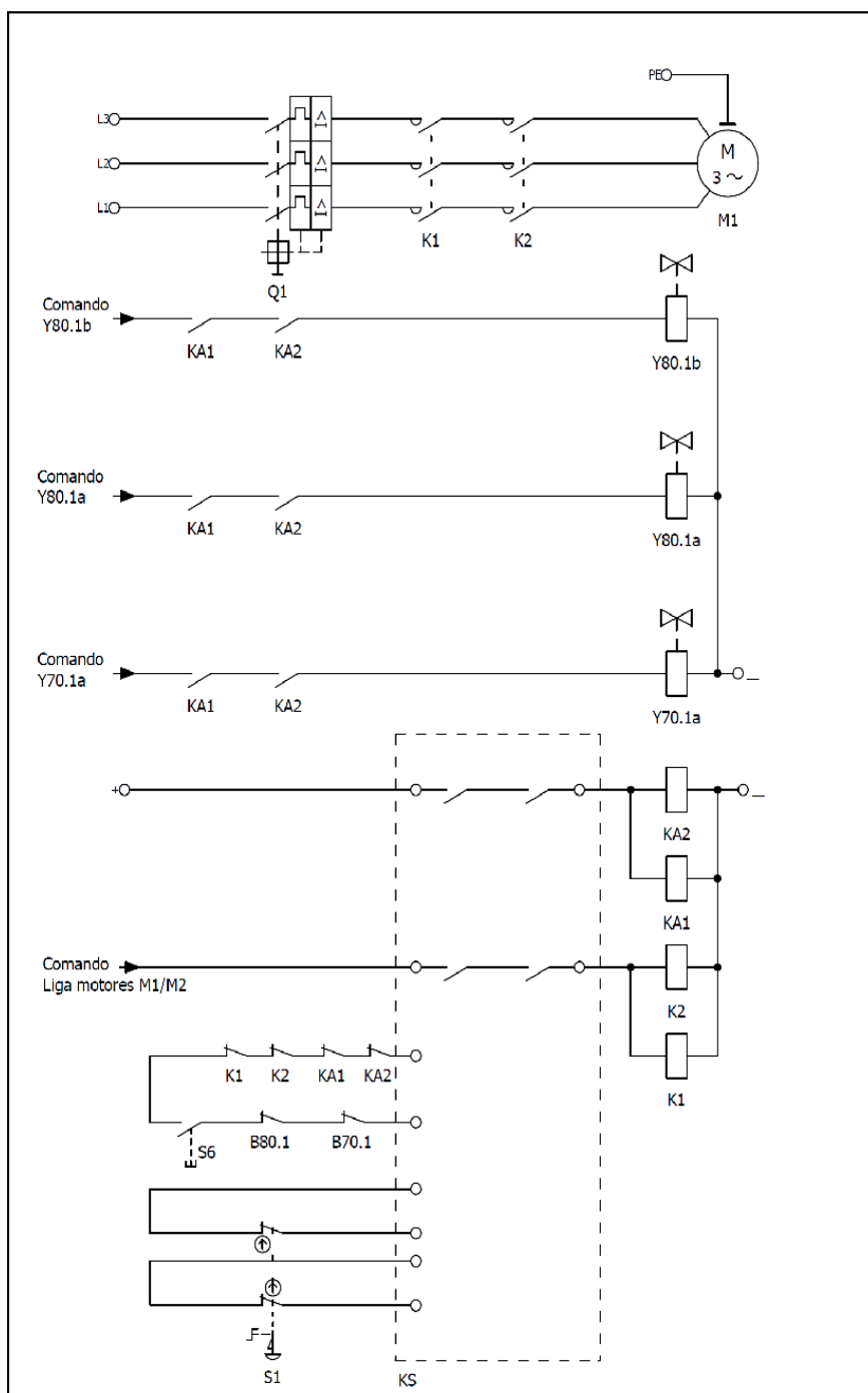
Figura 81: Circuito elétrico
