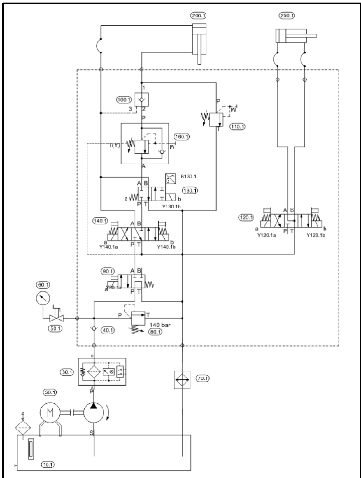
Figura 71: Circuito hidráulico
