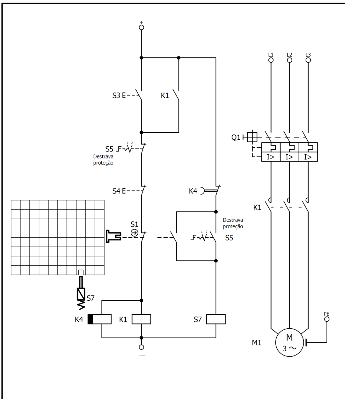
Figura 30: Circuito elétrico
