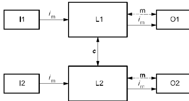
Figura 10: Categoria 3 - Fonte: ABNT NBR ISO 13849-1:2019
