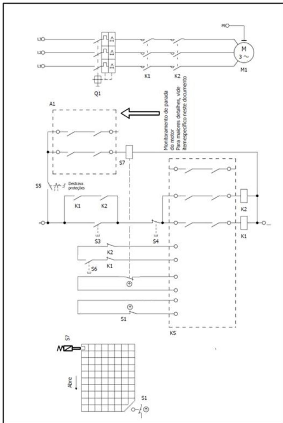
Figura 88: Circuito elétrico
