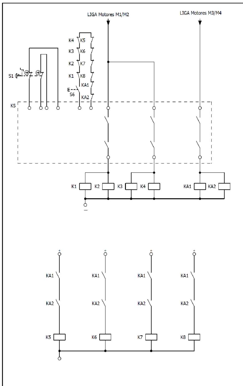
Figura 85: Circuito elétrico de comando
