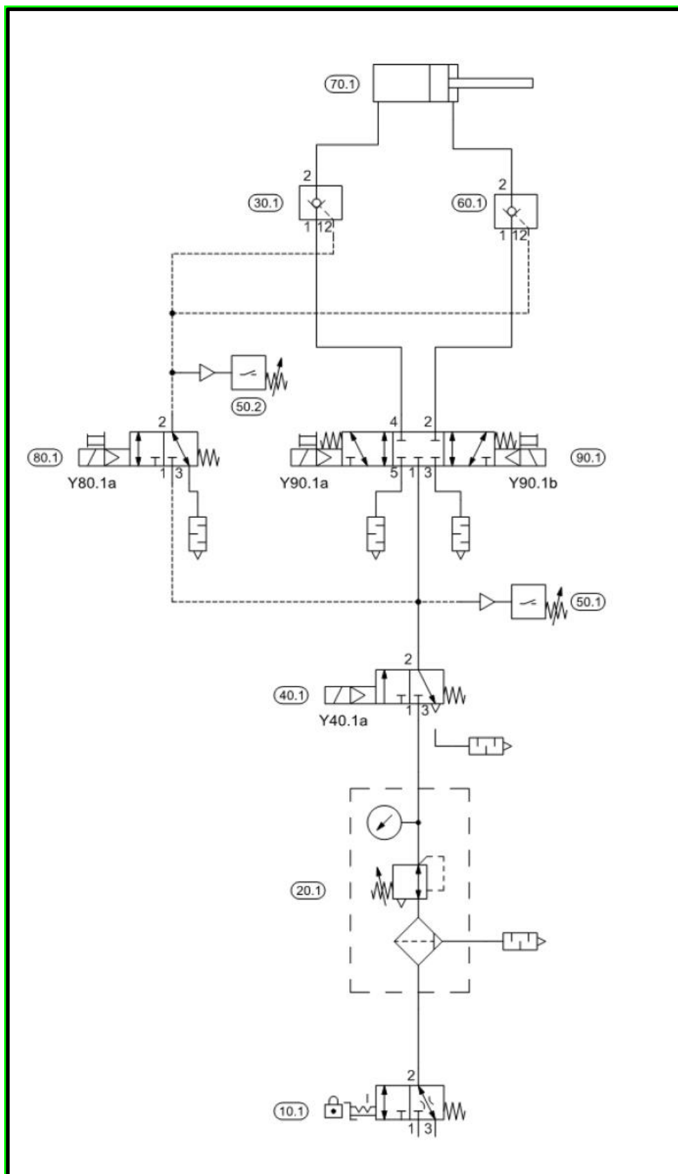
Figura 98: Circuito neumático
