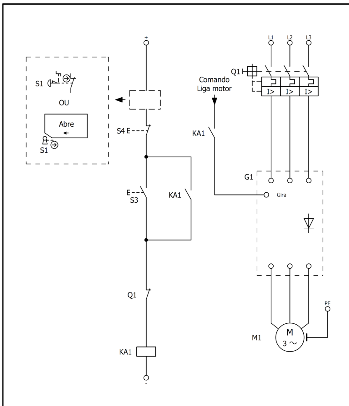
Figura 26: Circuito elétrico
