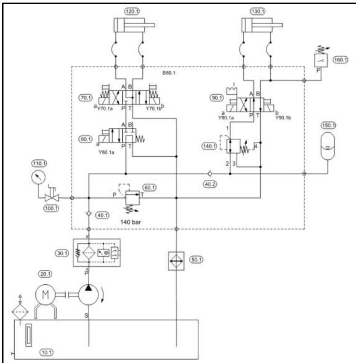
Figura 35: Circuito hidráulico
