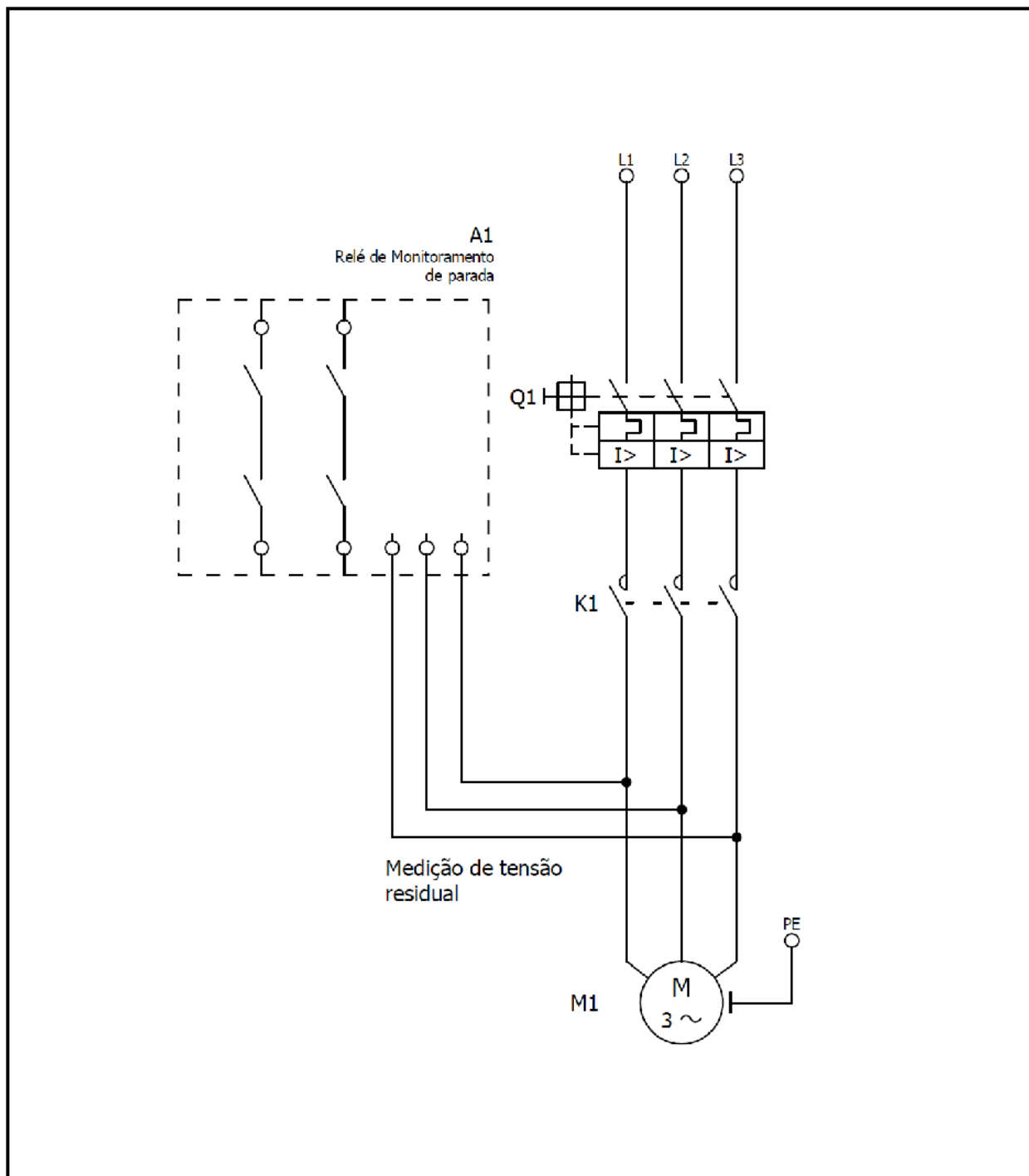
Figura 15: Circuito elétrico
