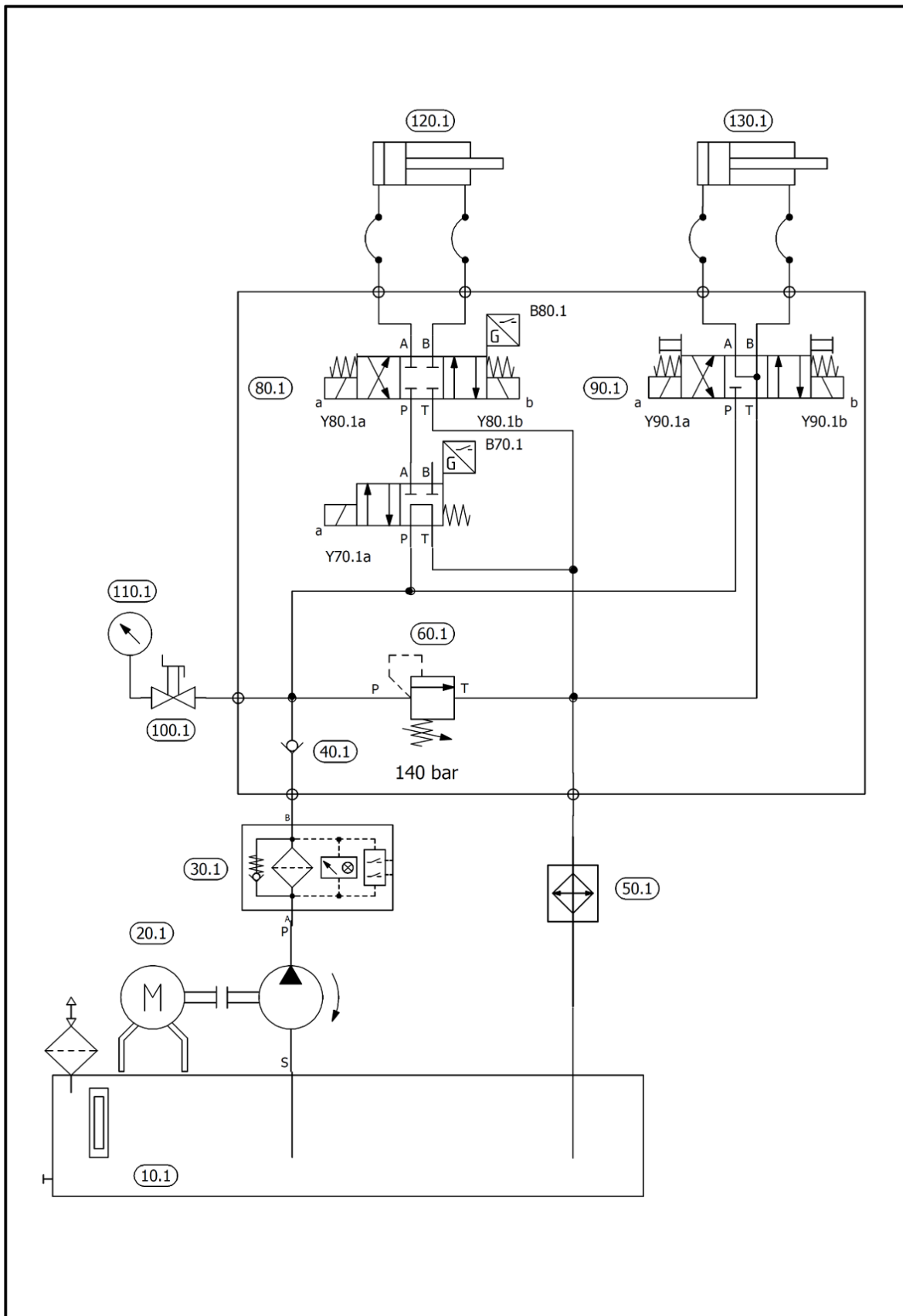
Figura 91: Circuito hidráulico
