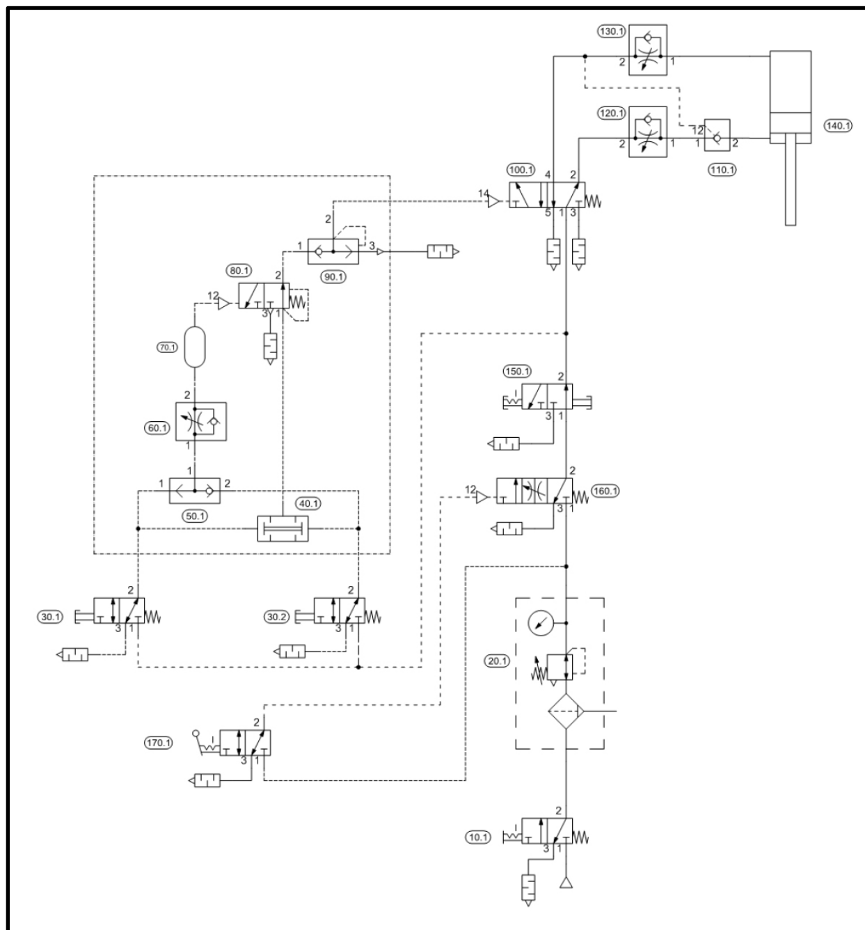
Figura 96: Circuito pneumático
