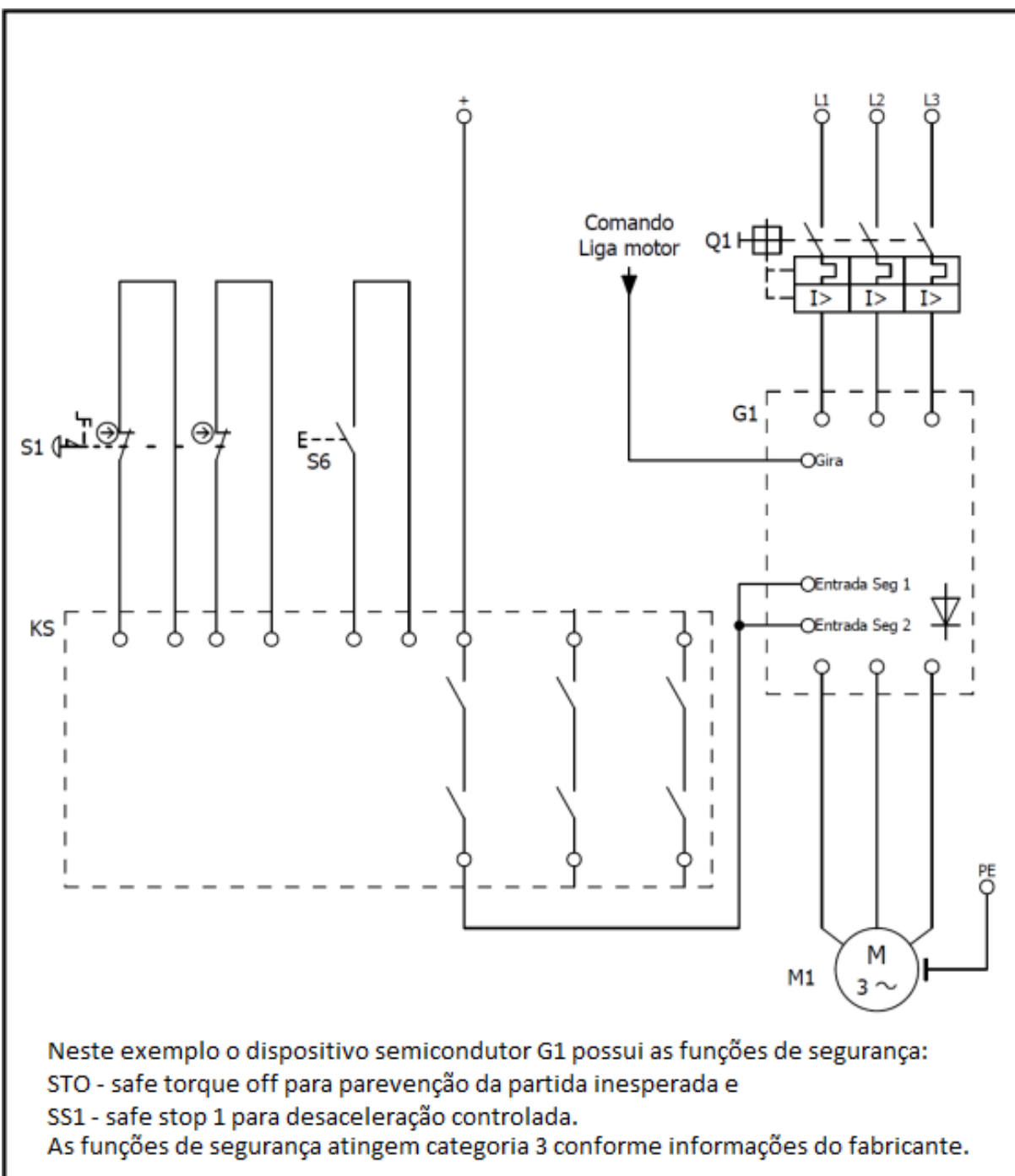
Figura 56: Circuito elétrico
