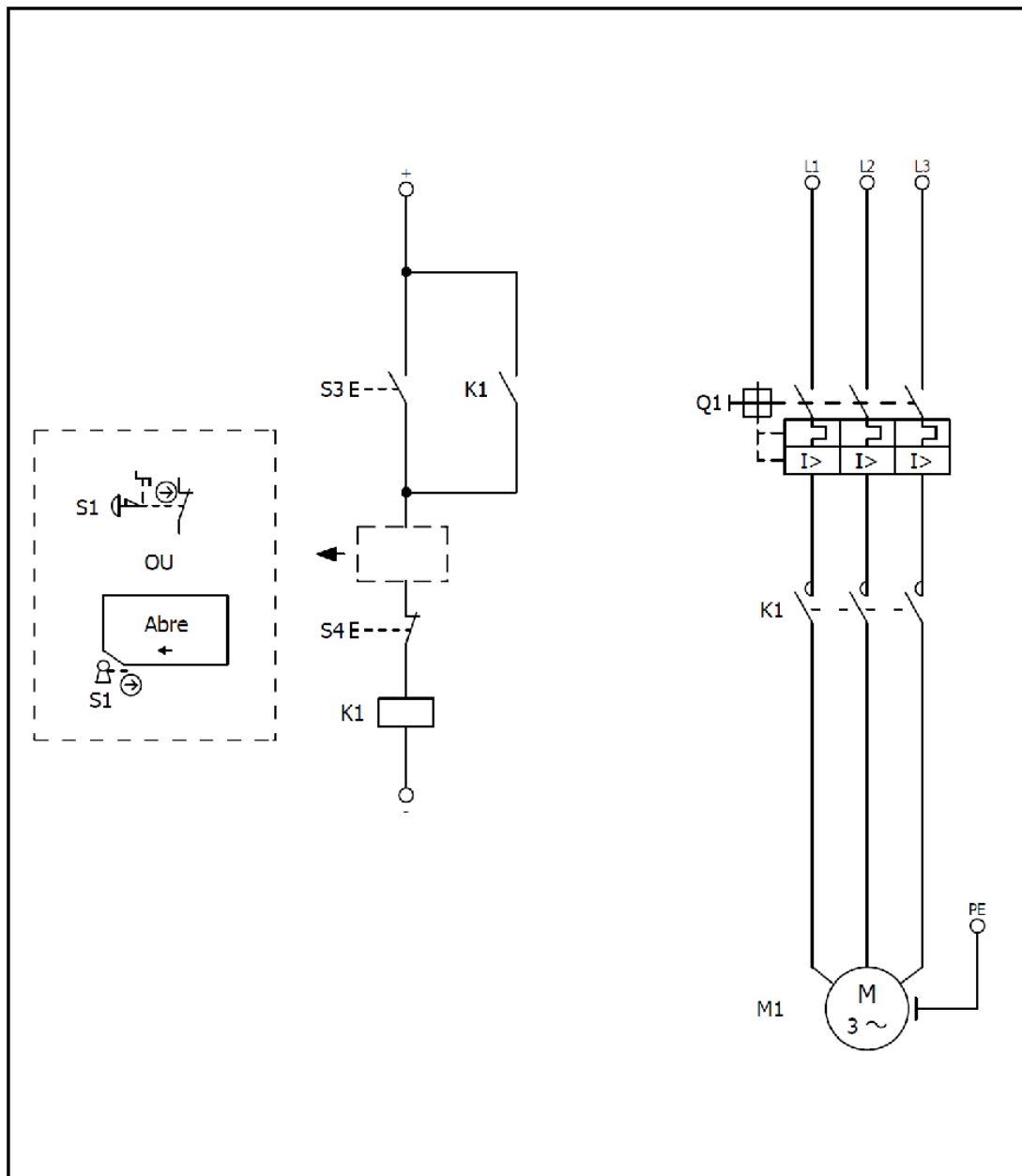
Figura 20: Circuito elétrico
