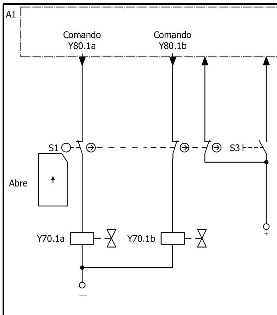
Figura 34: Circuito elétrico
