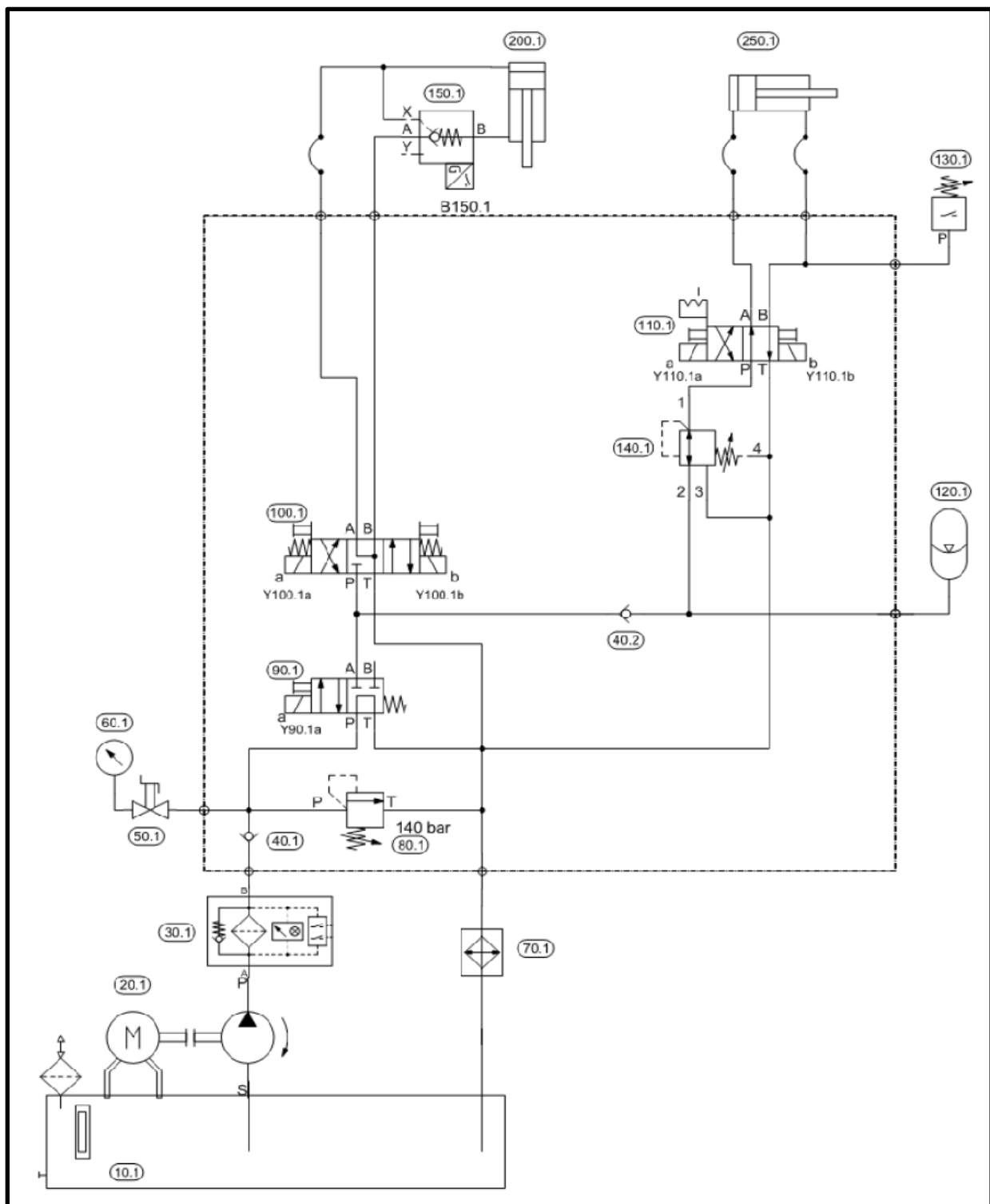
Figura 48: Circuito hidráulico
