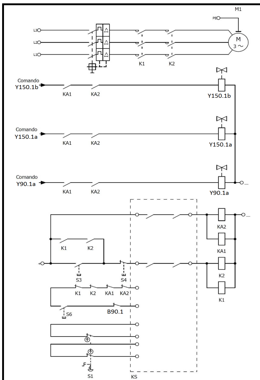
Figura 62: Circuito elétrico
