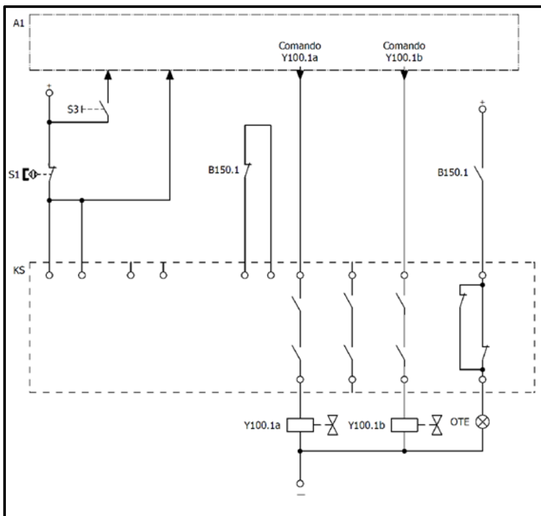
Figura 47: Circuito elétrico
