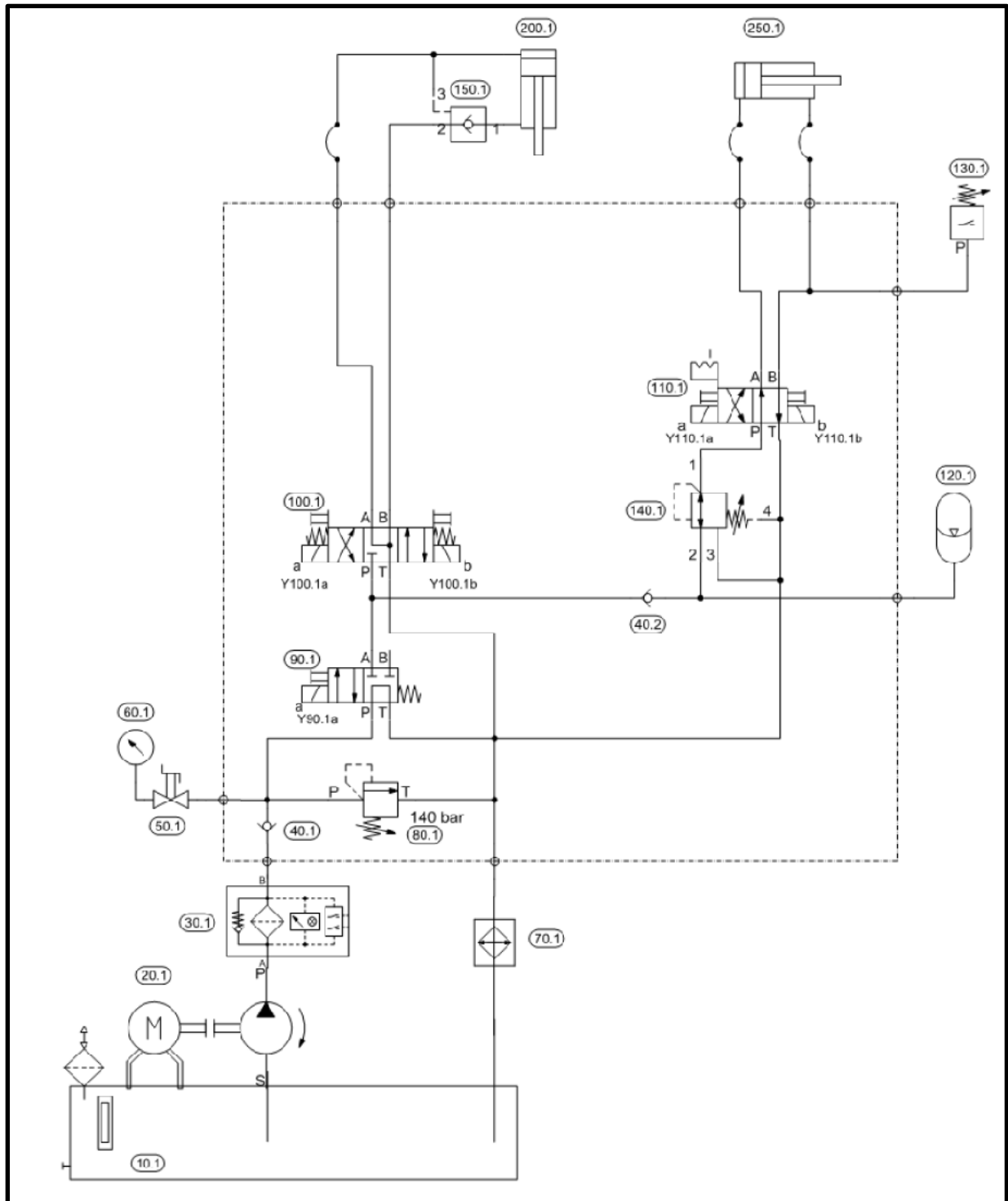
Figura 38: Circuito hidráulico
