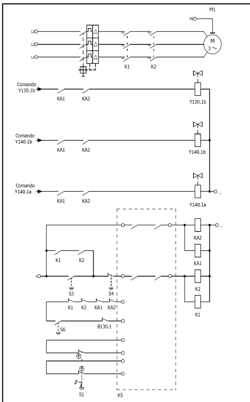
Figura 66: Circuito elétrico
