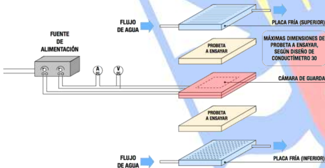
Figura N°1: Esquema montaje experimental
