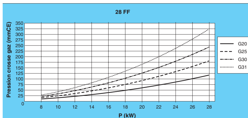
Graphe pression/puissance
