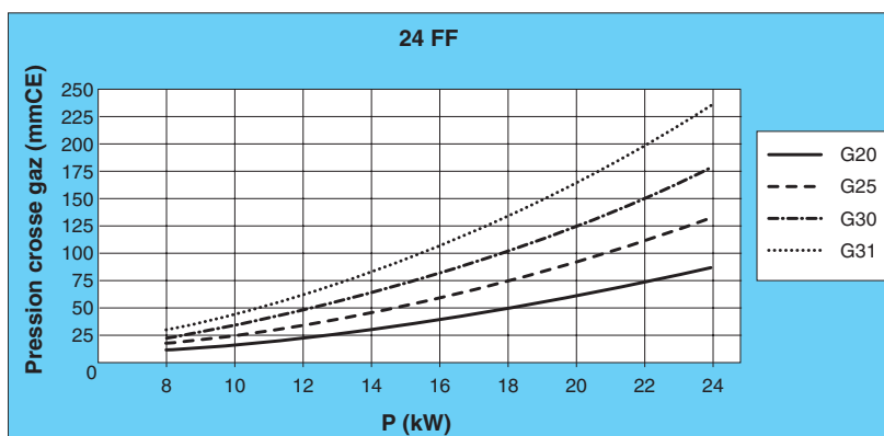
Graphe pression/puissance
