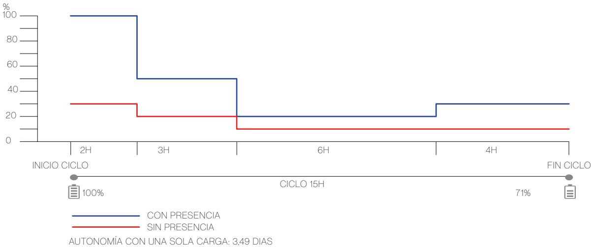
CURVA DE PROGRAMACIÓN Nº 1 (4 TRAMOS DE TIEMPO CON DETECCIÓN)
