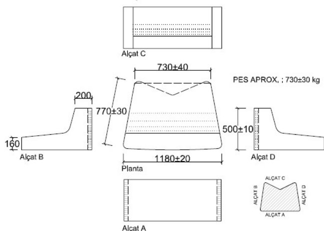
PEÇA CORONACIÓ
