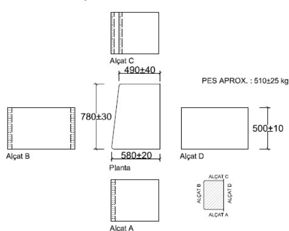
PEÇA CANTONADA
