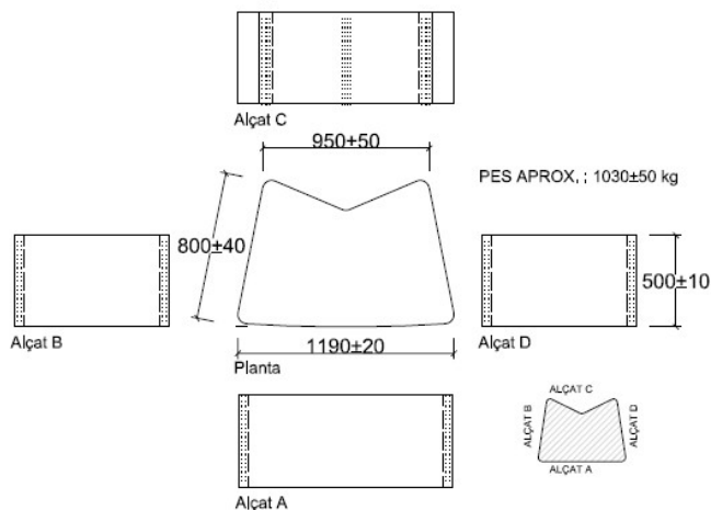
PEÇA SENCERA 1
