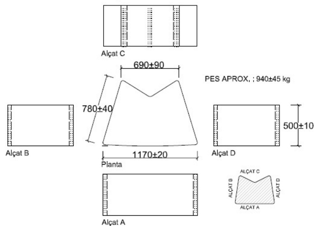
PEÇA SENCERA 2
