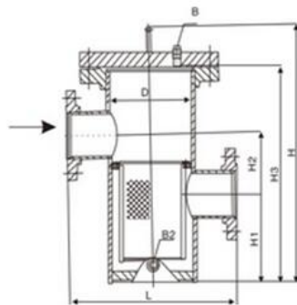
结构图
