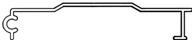
H136 Tapacinta 341 grs/mts Tiras por paquete: 10
