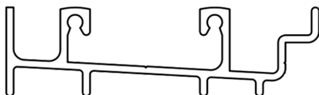
H112 Umbral puerta corrediza Transitable N°17 940 grs/mts Tiras por paquete: 4
