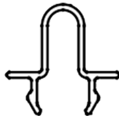
R313 Encuentro Tipo Rotonda 189 grs/mts Tiras por paquete: 10
