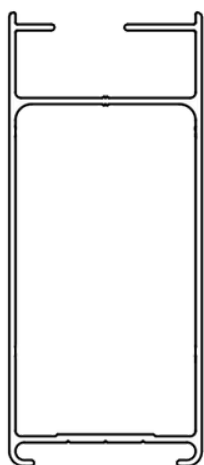
H118 Parante Puerta Hoja 36mm 972 grs/mts Tiras por paquete: 3
