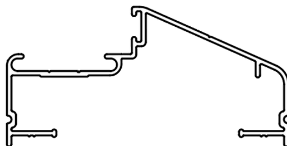
H117 Marco Puerta Hoja 25mm 456 grs/mts Tiras por paquete: 5
