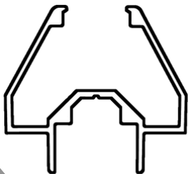
H157 Perimetral Liviano con Cava Espinosa 200 grs/mts Tiras por paquete: 10
