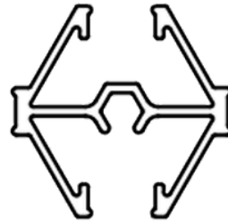
H152 Central con Cava Flamia 285 grs/mts Tiras por paquete: 10
