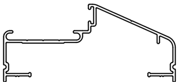
H116 Marco Puerta Hoja 36mm 521/mts Tiras por paquete: 5
