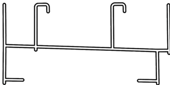
H109 N°1 Ala Ancha o Marco Recto 483 grs/mts Tiras por paquete: 6
