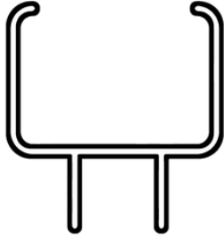
H126 Doble Vidriado 255 grs/mts Tiras por paquete: 10
