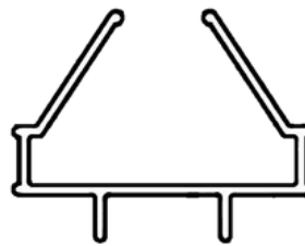
H156 Perimetral Liviano sin Cava Flamia 198 grs/mts Tiras por paquete: 10
