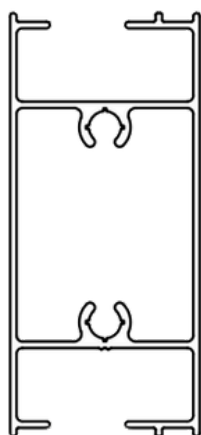
H120 Travesaño Puerta Hoja 36mm 1000 grs/mts Tiras por paquete: 3
