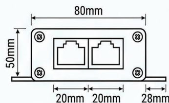
RS-485 (Modbus)
